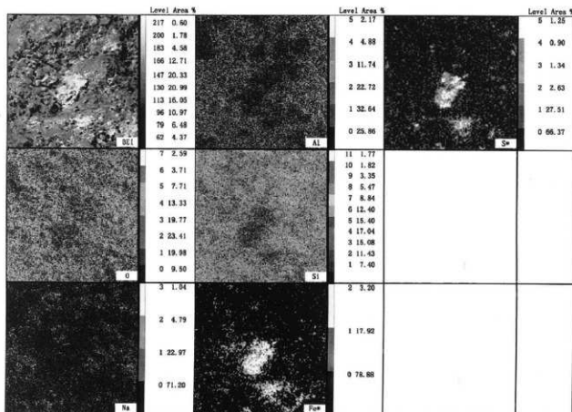
EDX分析図
