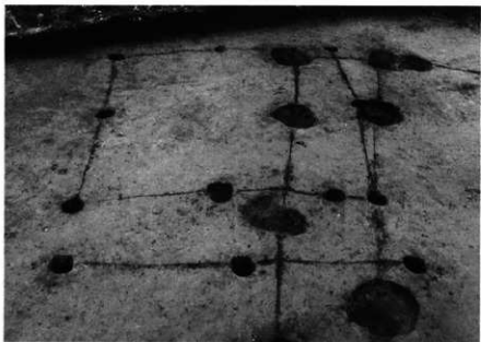
第24図 F-6号掘立柱建物址
