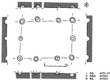
第11图 F-2号掘立柱建物址 (1:80)
