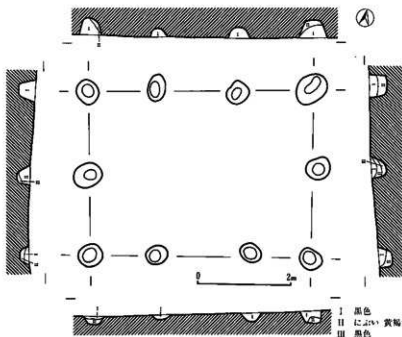
第13図 F-4号掘立柱建物址 (1:80)
