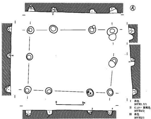
第14图 F-5号独立柱建物址 (1:80)
