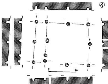
第15图 F-6号独立柱建物址 (1:80)
