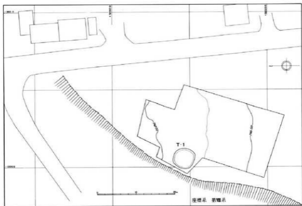
第3図 前廊部遺跡全体図 (1 : 500)
