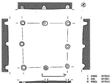
第10图 F-1号掘立柱建物址 (1:80)
