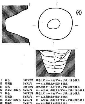
第18図 D-1号土坑実測図 (1:80)
