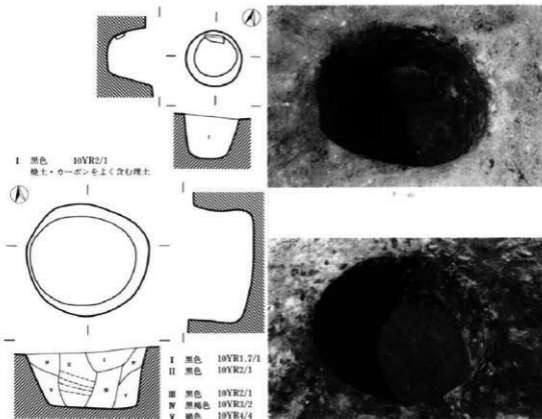
第7図 上ノ屋敷遺跡D-1(上)・D-2(F)(1:40)
