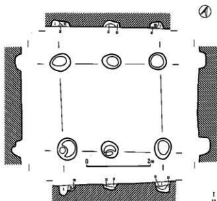
第12図 F-3号掘立柱建物址 (1:80)
