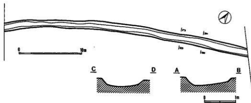
第19図 M-1号溝状遺構実測図 (1:300)
