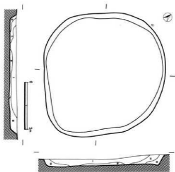
第5图 T-1号竖穴状遗构实测图 (1:80)
