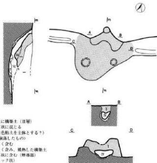
第7図 H-1号住居址カマド (1:40)
