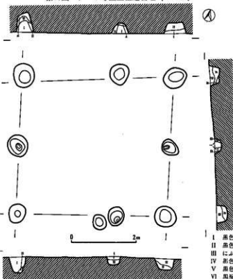
第16图 F-7号掘立柱建物址 (1:80)
