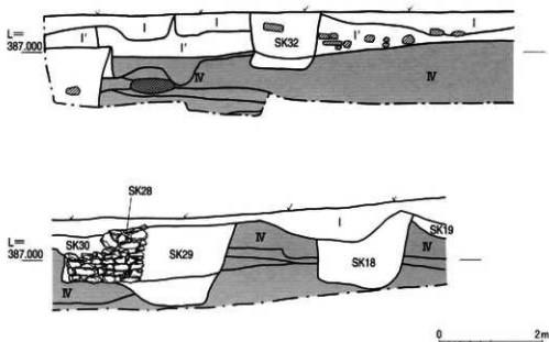
図4 試掘トレンチ南壁土層堆積断面(1:80)
