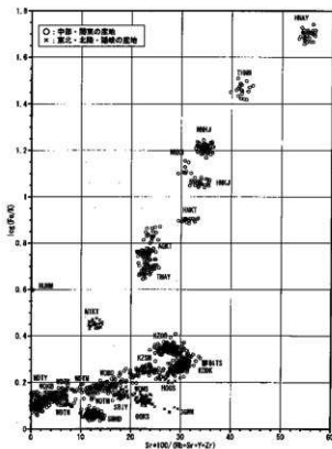
第43図 旧検出器による東日本・關東の産地原石判別図
