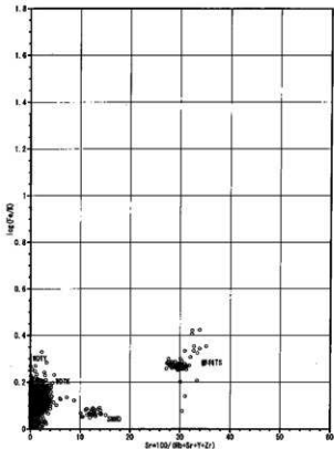
第44図 日向林B遺跡出土黒曜石の産地判別図
