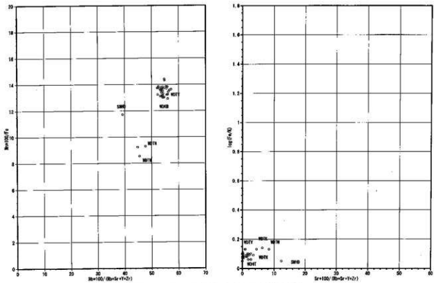
第47図 セン栗遺跡出土黒曜石の産地判別図
