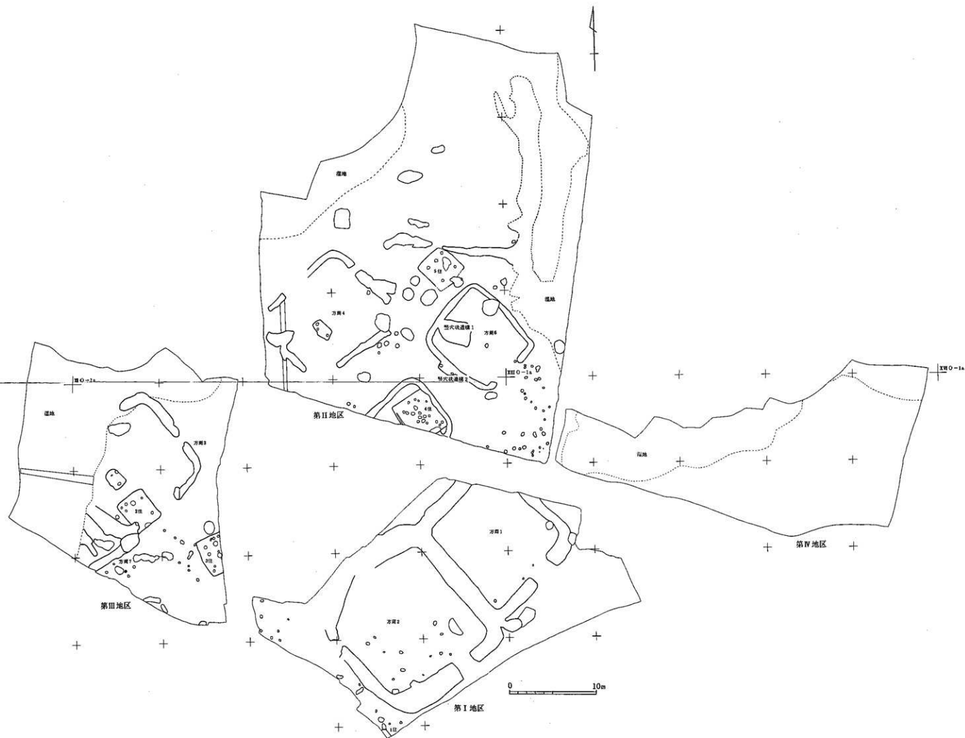
付图3 橘爪遺跡第I・II・III・IV地区全体图(1:300)
