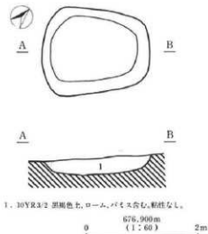
第8図 D2号土坑実測図
