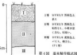
第4図 基本層序模式図
