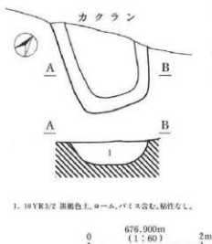
第7図 D1号土坑実測図
