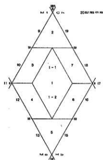
第57図 菱形ダイアグラム位置分類図
