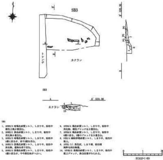
第24図 SB3 実測図
