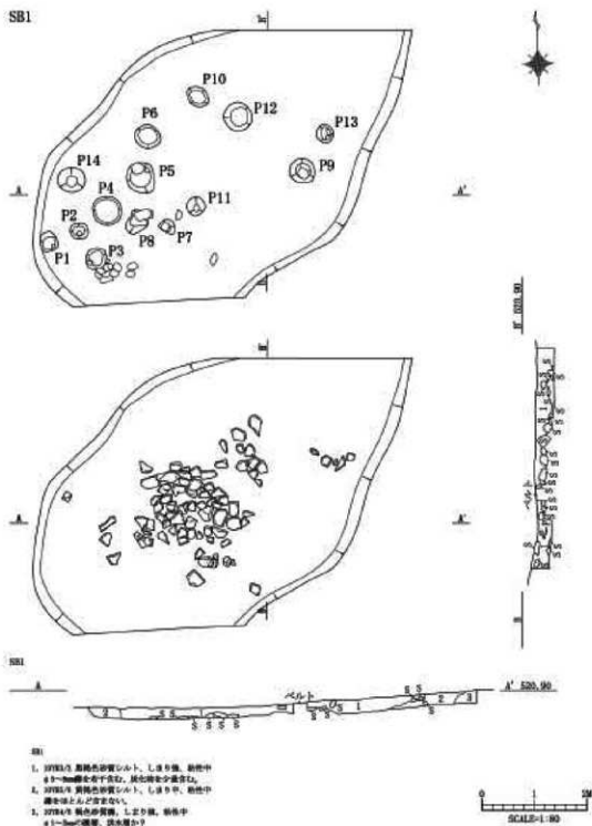
第22図 SB1実測図
