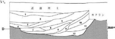
第6図 溝状遺構土層断面図 (1:80)
