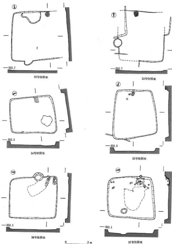
156图 L区住居址实测图(52号·53号·54号·55号·56号·57号)
