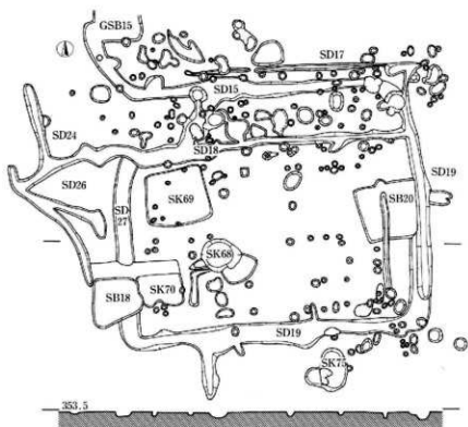
周溝內柱穴群·土壤群 (1:250)
