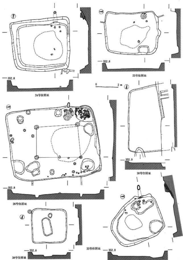
131图 丁区住居址实测图 (24号·25号·26号·30号·33号·38号)
