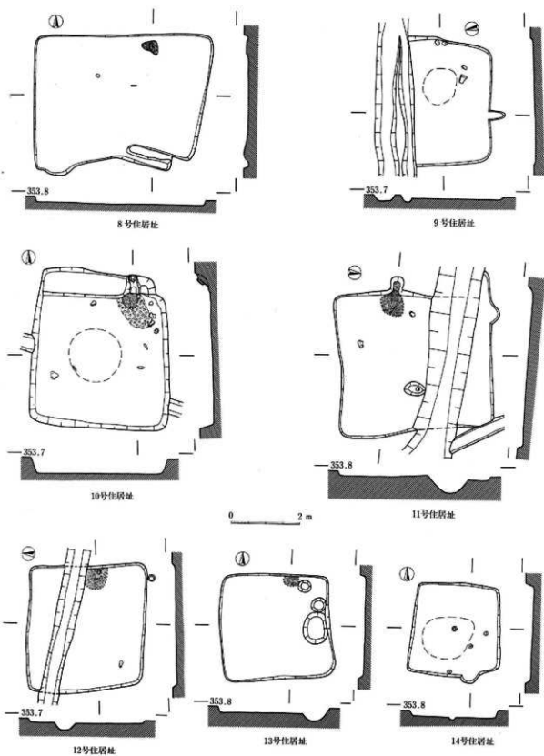
150图 L区住居址实测图(8号·9号·10号·11号·12号·13号·14号)
