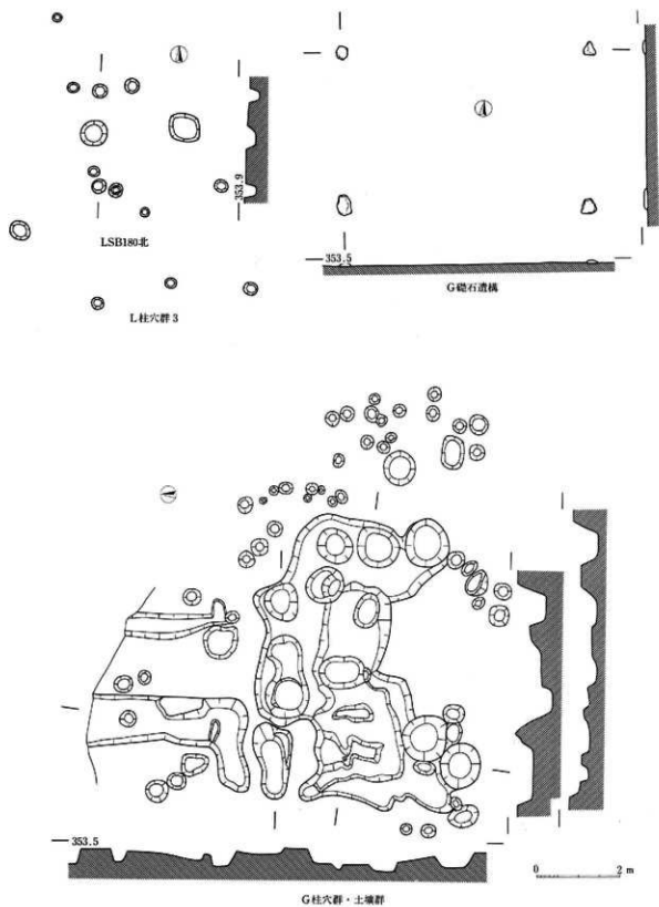
180图 L·G区柱穴群、G区礎石遺構・柱穴群・土壇群実測图 (1:100)
