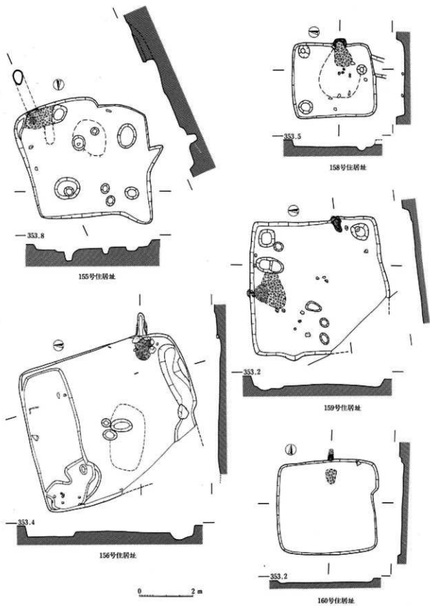
170图 L区住居址实测图(155号·156号·158号·159号·160号)
