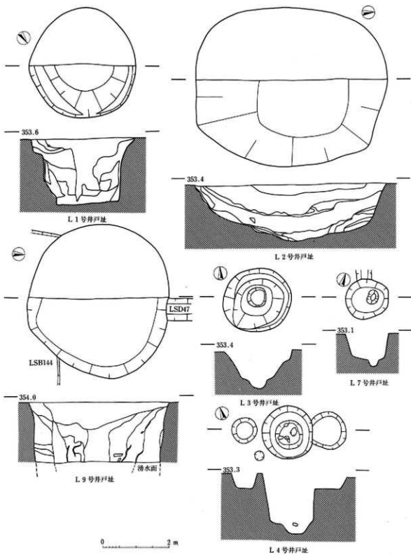
182图 L区井尸址实测图 (L区1~4·7·9号)
