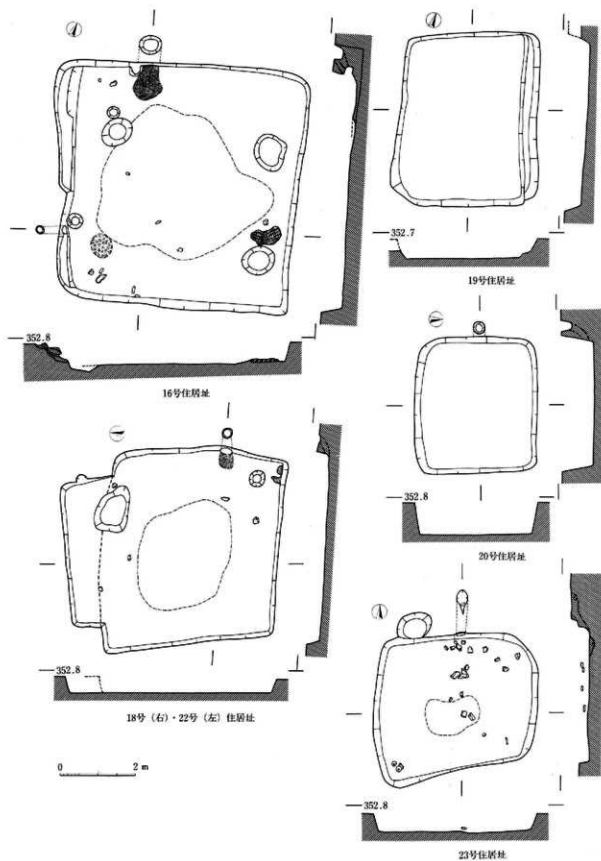
127图 丁区住居址实测图(16号·18号·19号·20号·22号·23号)
