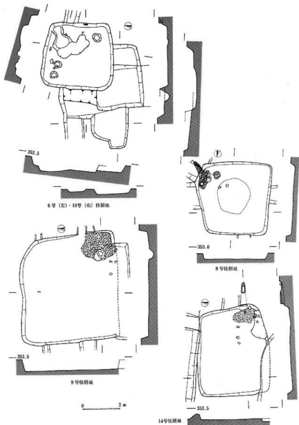
134图 K区住居址实测图(6号·8号·9号·10号·14号)
