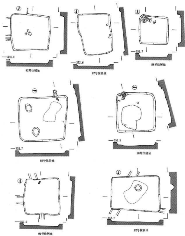
145图 K区住居址实测图 (82号·87号·88号·89号·90号·91号·92号)
