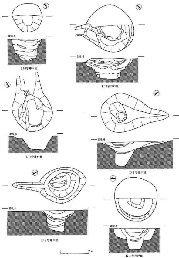
181图 D·K·L区井尸址实测图
