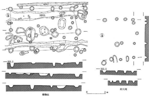
177图 G区周溝內柱穴群(建物址·柱穴列)·土壤群实测图(1:100)
