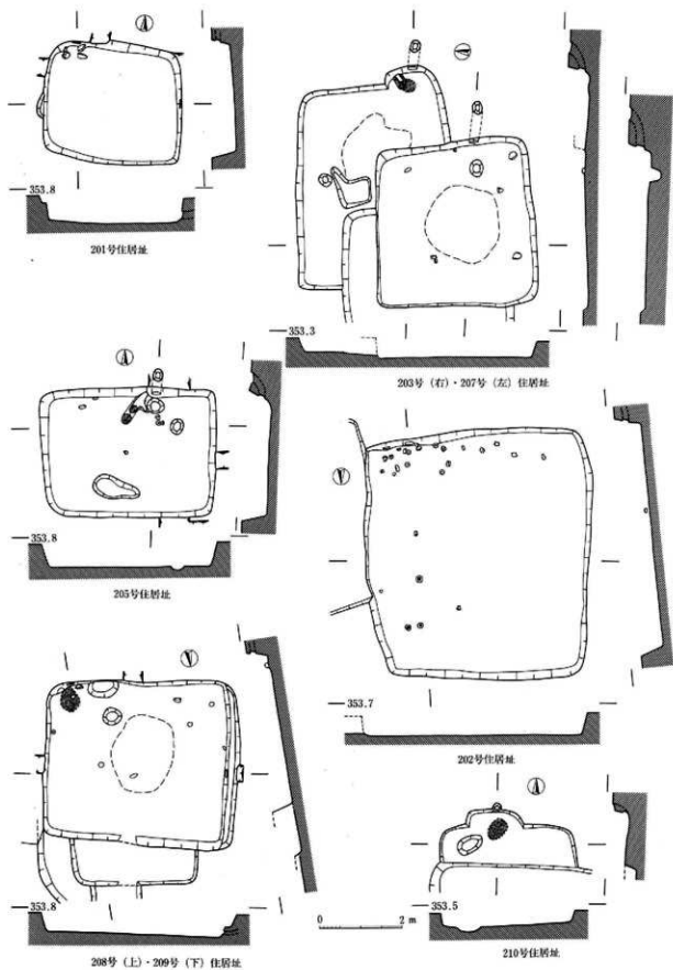
97图 I区住居址实测图(201号·202号·203号·205号·207号·208号·209号·210号)
