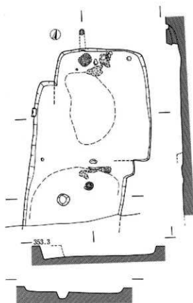
193号(下)·195号(上)住居址
