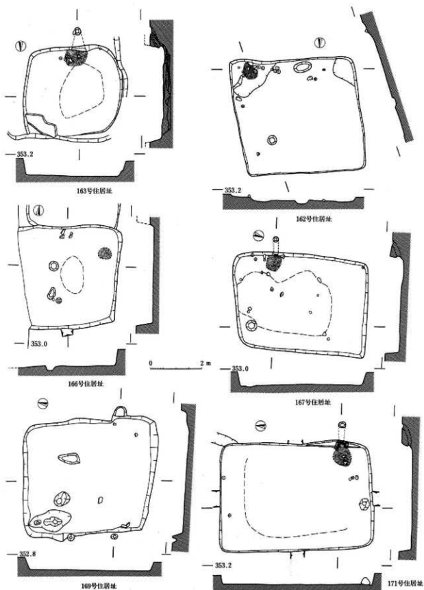
122图 I区住居址实测图(162号·163号·166号·167号·169号·171号)
