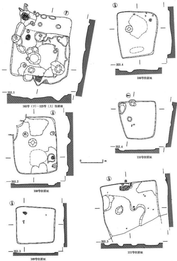
90图 1区住居址实测图(103号·106号·108号·109号·110号·111号·125号)
