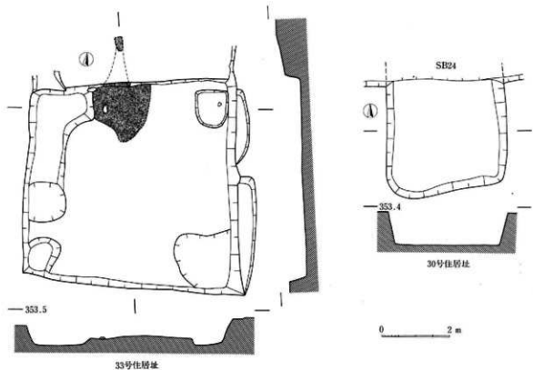
75图 G区住居址实测图(27号·30号·31号·33号)
