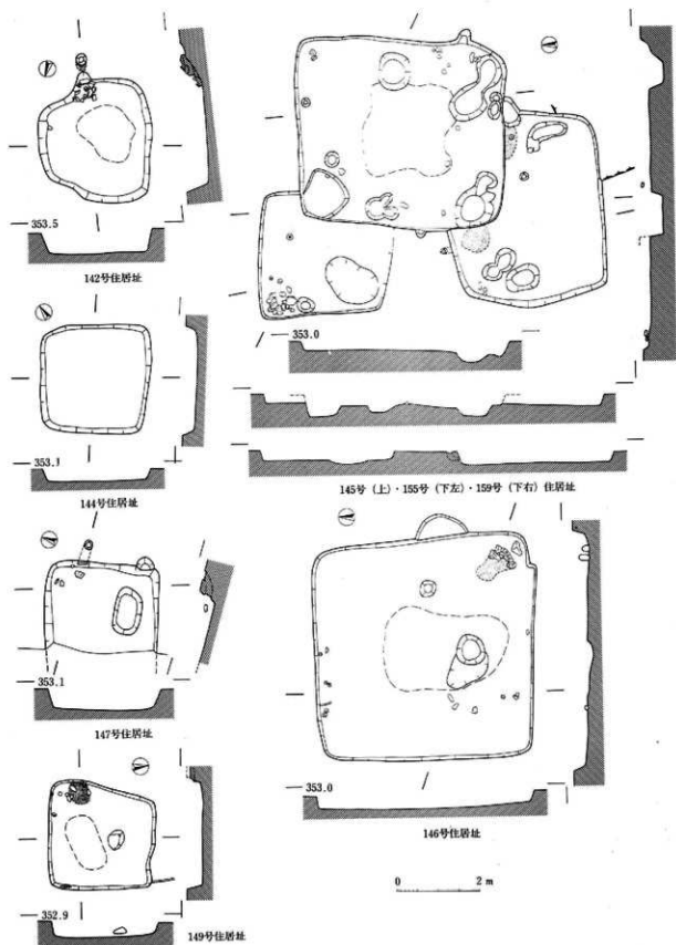
119图 I区住居址实测图(142号·144号·145号·146号·147号·149号·155号·159号)
