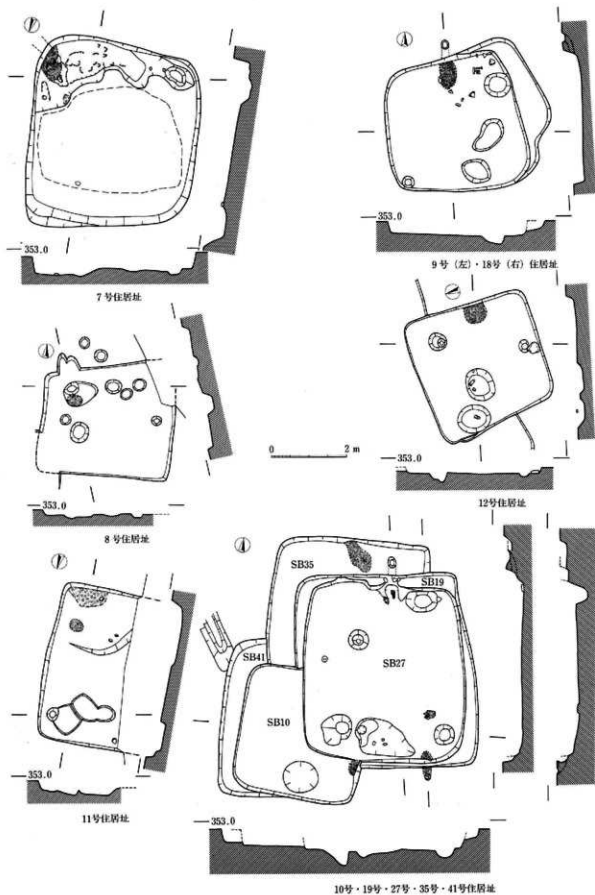
114图 I区住居址实测图(7号·8号·9号·10号·11号·12号·18号·19号·27号·35号·41号)
