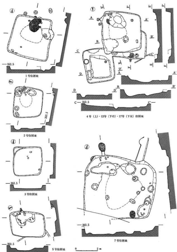
85图 H区住居址实测图(1号·2号·3号·4号·5号·7号·13号·17号)
