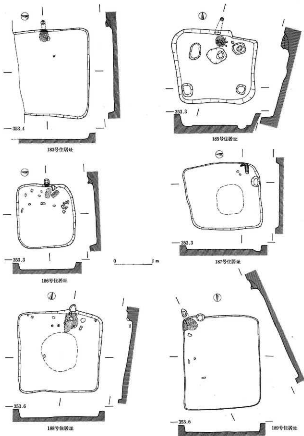
94图 I区住居址实测图 (183号·185号·186号·187号·188号·189号)
