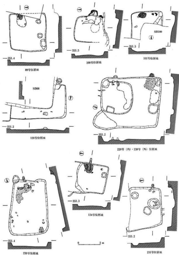
105图 I区住居址实测图(89号·100号·101号·120号·124号·220号·230号·231号·238号)
