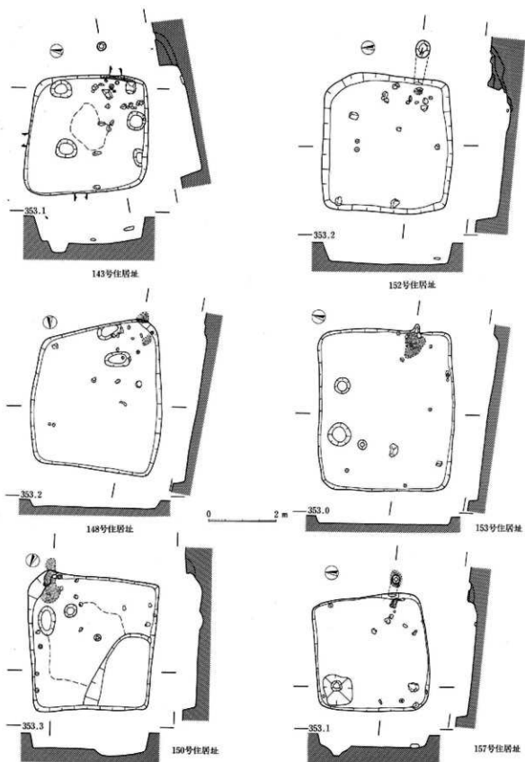
120图 I区住居址实测图 (143号·148号·150号·152号·153号·157号)
