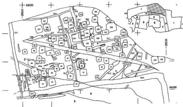
99図 第IV群I区(中)・E・H区遺構分布図(1:800)
