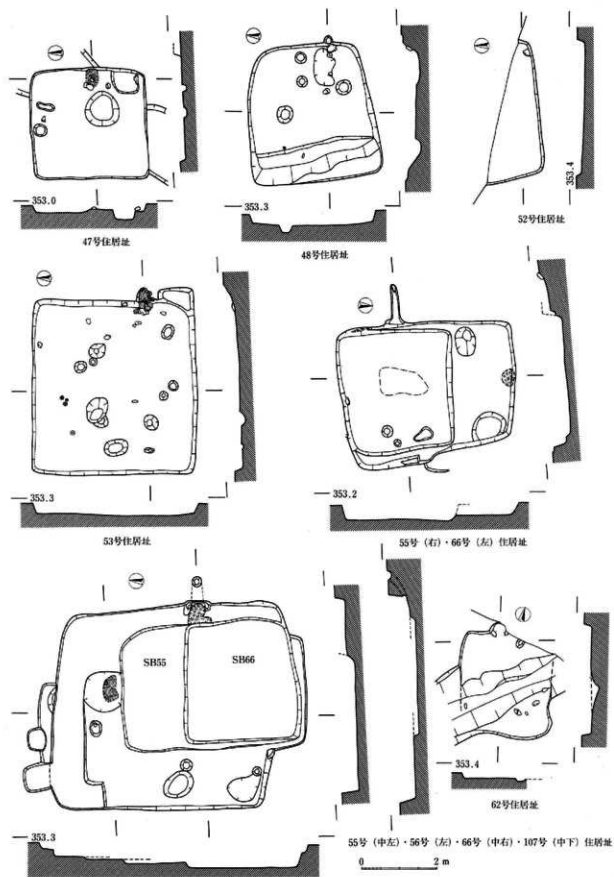
101图 I区住居址实测图(47号·48号·52号·53号·55号·56号·62号·66号·107号)
