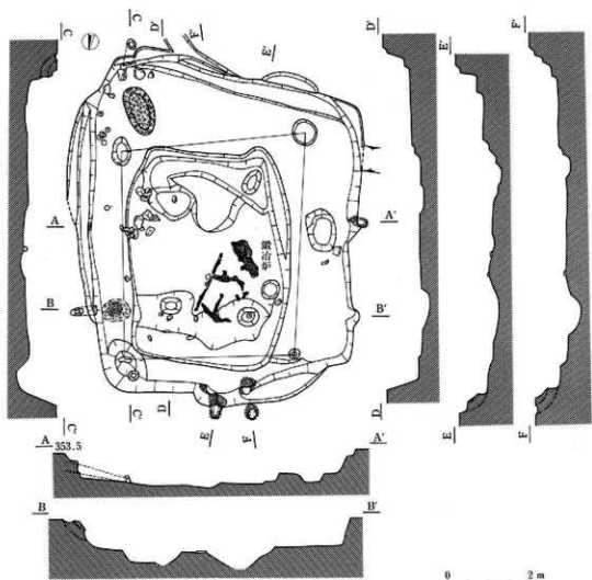
41号(外)·43号(中)住居址
