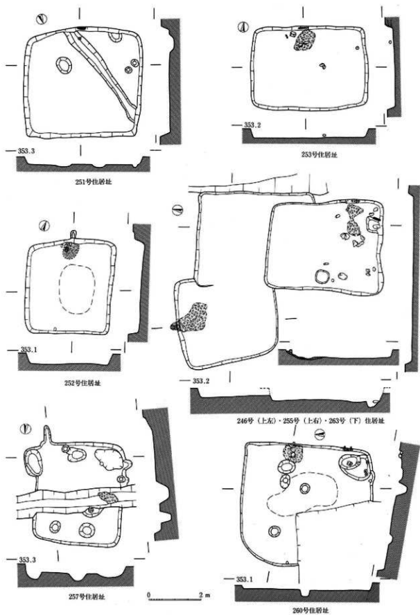
109图 I区住居址实测图(246号·251号·252号·253号·255号·257号·260号·263号)
