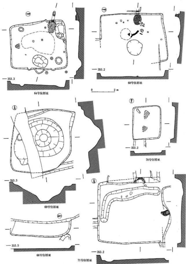
81图 H区住居址实测图 (64号·66号·68号·69号·70号·71号)
