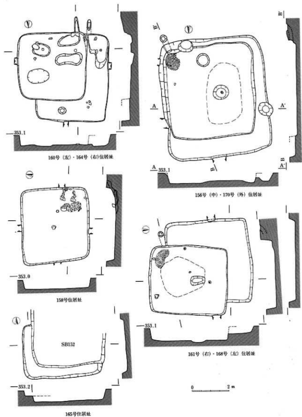
121图 I区住居址实测图(156号·158号·160号·161号·164号·165号·168号·170号)
