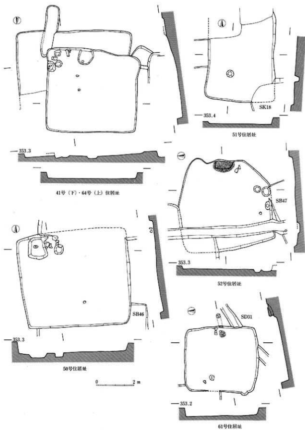
66图 F区住居址实测图(41号·50号·51号·52号·61号·64号)
