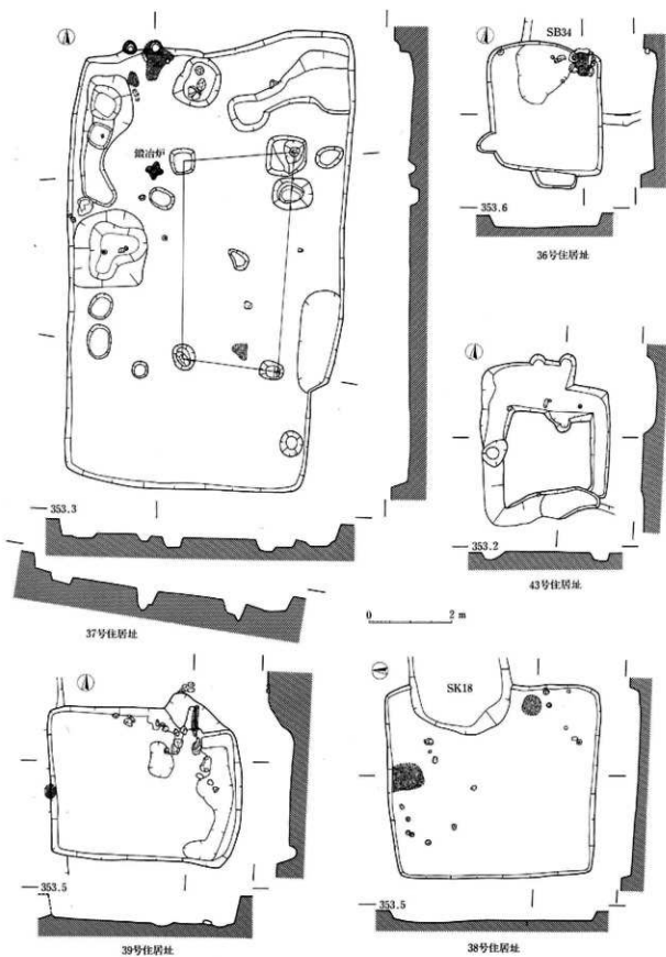
64图 F区住居址实测图(36号·37号·38号·39号·43号)
