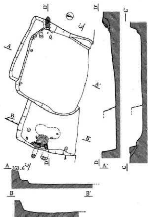
194号(上)·204号(下)住居址
