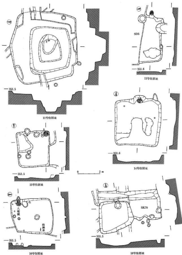
70图 G区住居址实测图 (11号·13号·14号·15号·16号·18号)
