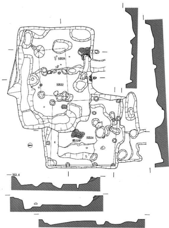
28号(上)·32号(中)·34号(下)住居址
