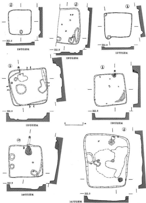
118图 I区住居址实测图(135号·136号·137号·138号·139号·140号·141号)
