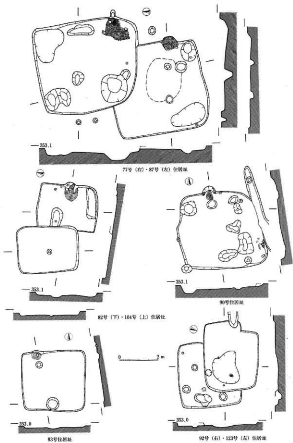
88图 I区住居址实测图(77号·82号·87号·90号·92号·93号·104号·123号)
