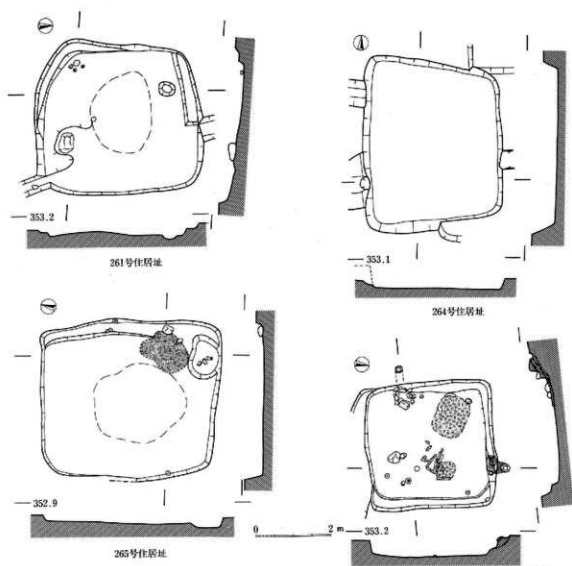
111图 I区住居址实测图(261号·264号·265号·266号)
