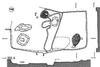
38号(右)·42号(左)住居址
