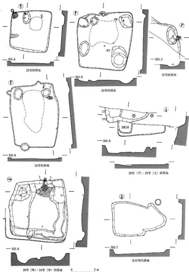
100图 H区(22号·24号·25号·29号·31号·33号·34号)·E区(37号)住居址实测图
