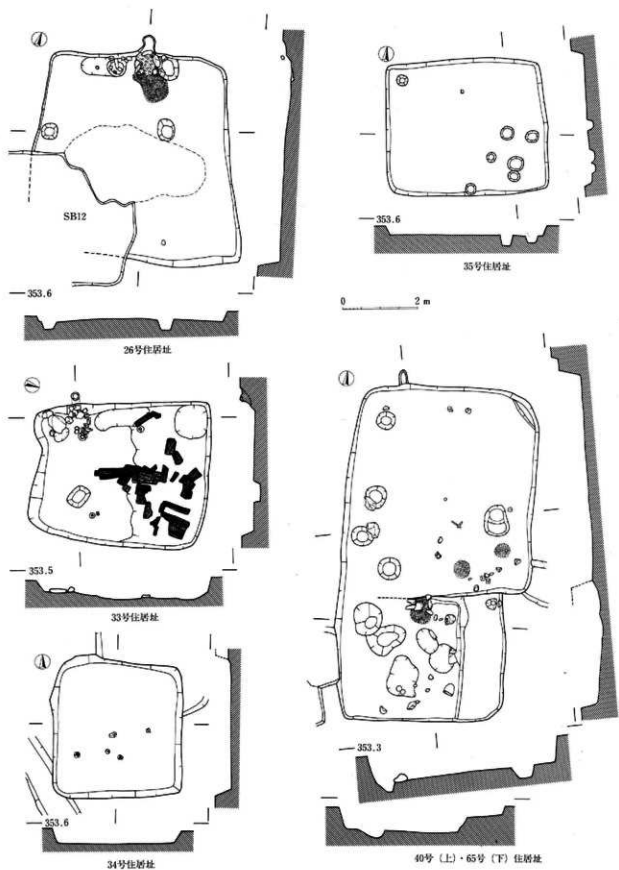
63图 F区住居址实测图(26号·33号·34号·35号·40号·65号)
