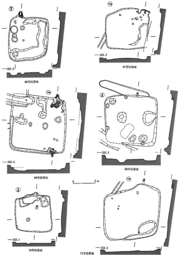
103图 I区住居址实测图(60号·67号·68号·69号·70号·71号)
