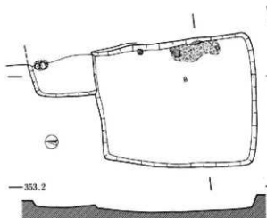
40号(右)·49号(左)住居址
