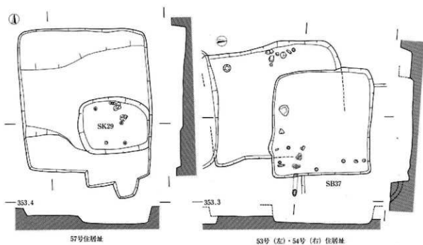
67图 F区住居址实测图(45号·53号·54号·57号·58号)
