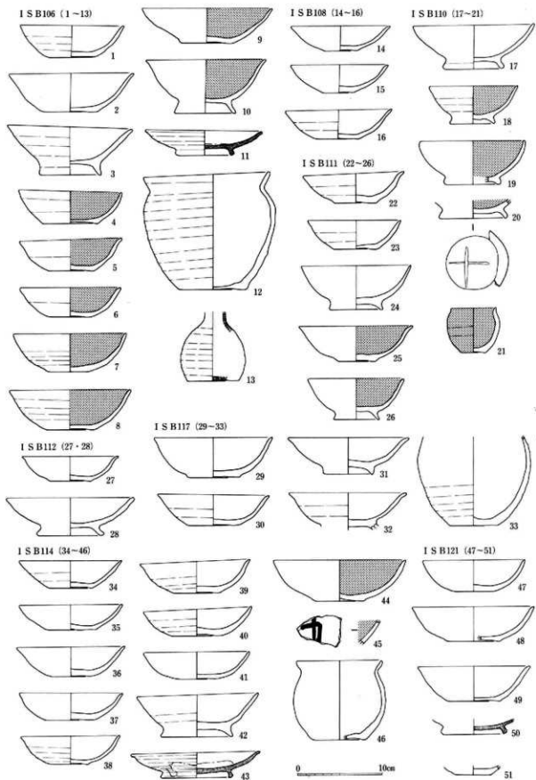
151图 I S B 106 · 108 · 110 ~ 112 · 114 · 117 · 121出土土器实测图 (1 : 4)
