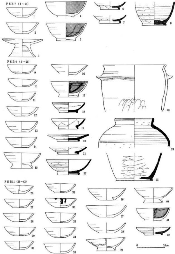
82图 FSB 7·9·11出土土器实测图(1:4)
