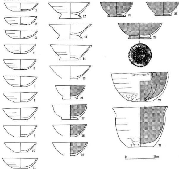
131図 HS B37・39出土土器実測図 (1:4)
