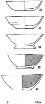
129图 HSB27·30·31·35·36·38·40·43出土土器实测图(1:4)
