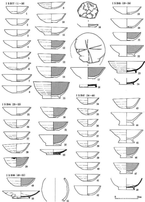
149图 I S B77·84·85·87·90出土土器实测图 (1:4)
