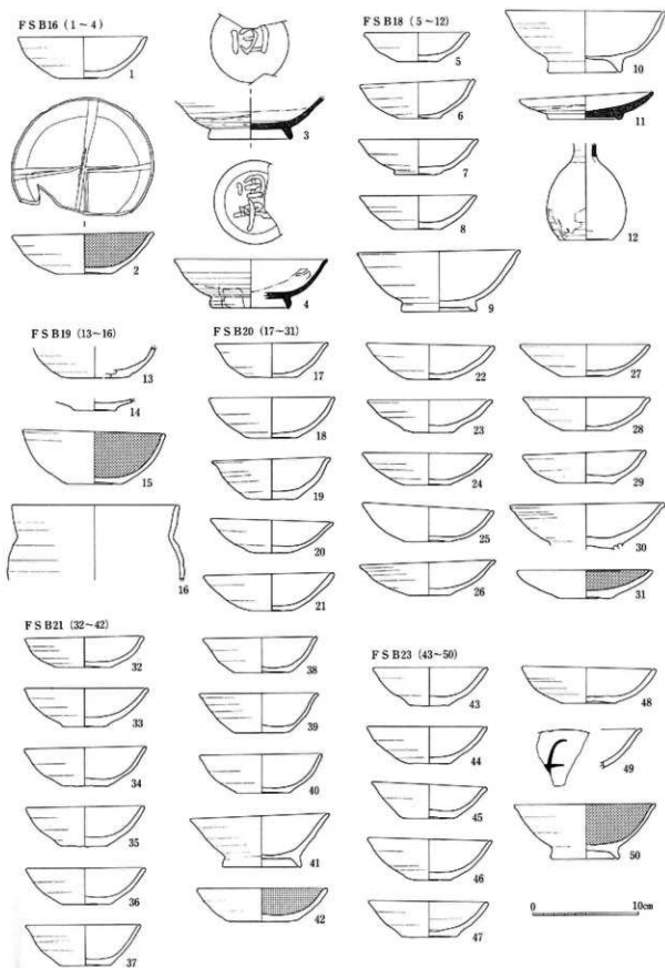
86图 FSB16·18~21·23出土土器实测图(1:4)
