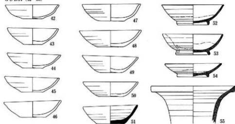
128图 GSB31·34出土土器实测图(1:4)
