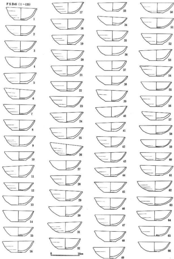
96图 FSB45出土土器实测图(1:4)
