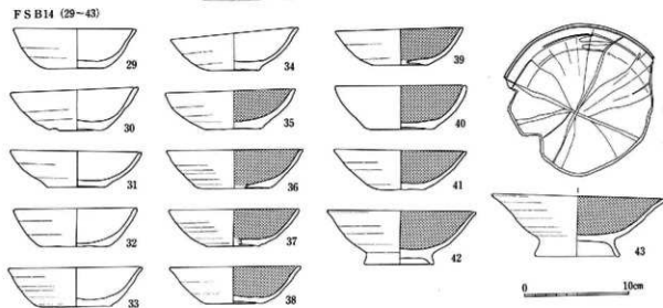
83图 FSB10·13·14出土土器实测图(1:4)
