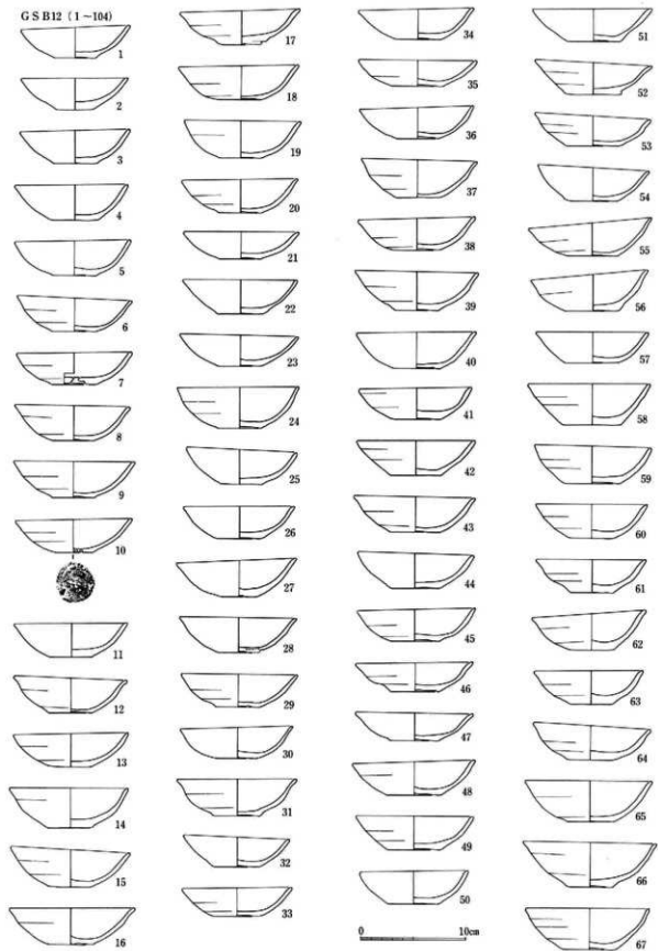
111图 GS B12出土土器实测图 (1:4)
