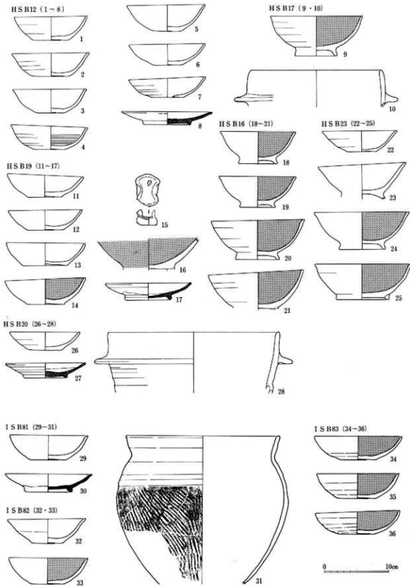
148圖 HS B12・16・17・19・20・23, IS B81~83出土土器実測図(1:4)
