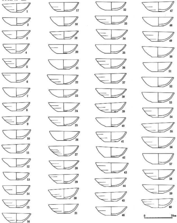
125図 G S B27・28出土土器実測図 (1 : 4)
