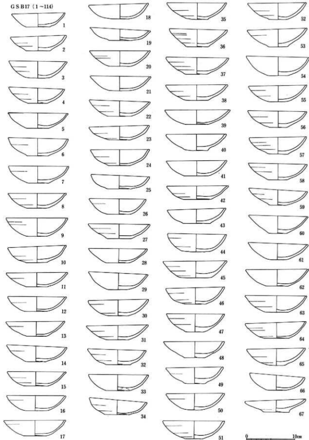
115图 GSB17出土土器实测图(1:4)
