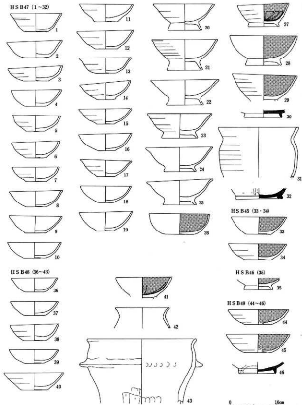
133图 HS B45~49出土土器实测图(1:4)
