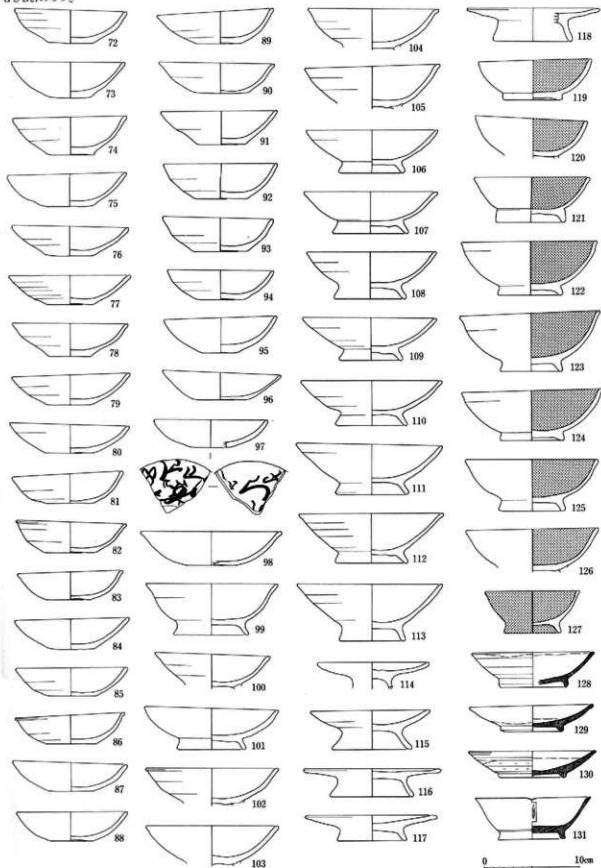
124図 GSB27出土土器実測図(1:4)
