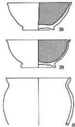
143图 I S B 45·46·51·61出土土器实测图(1:4)
