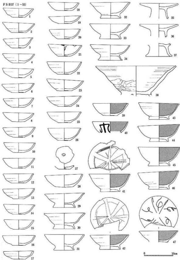
92图 FS B37出土土器实测图 (1:4)
