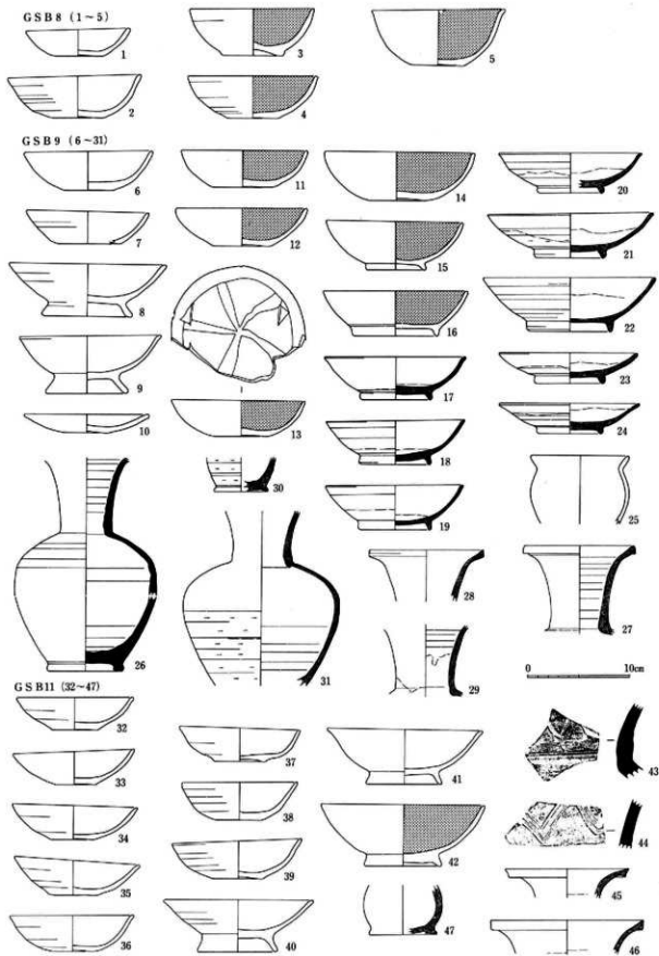
109图 GSB 8·9·11出土土器实测图(1:4)
