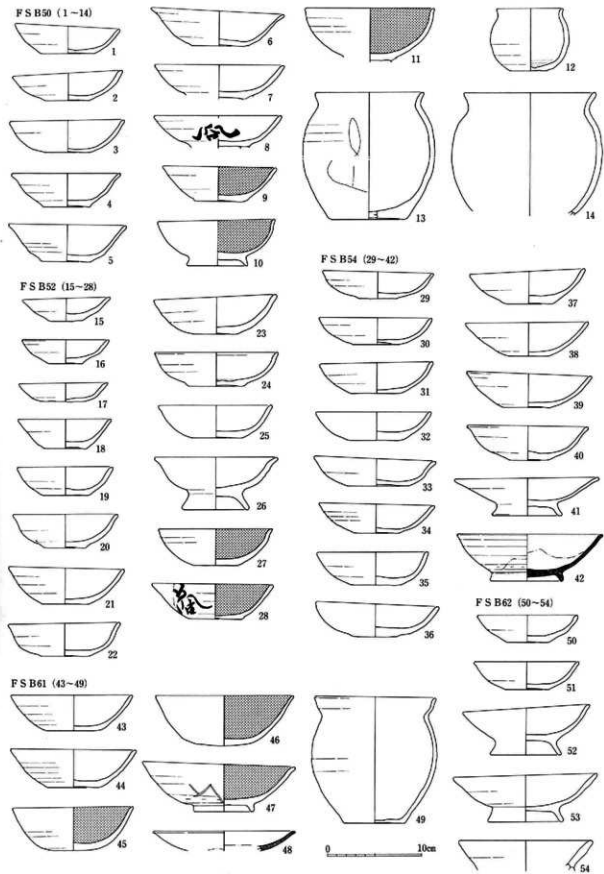
102图 FSB 50·52·54·61·62出土土器实测图(1:4)
