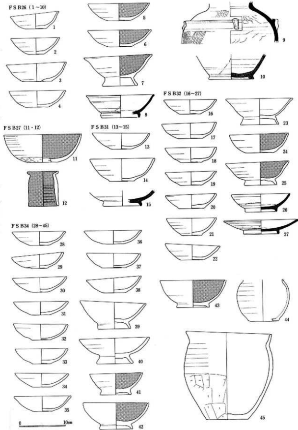
88图 FS B26·27·31·32·34出土土器实测图(1:4)
