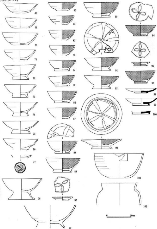
112図 GSB12出土土器実測図(1:4)
