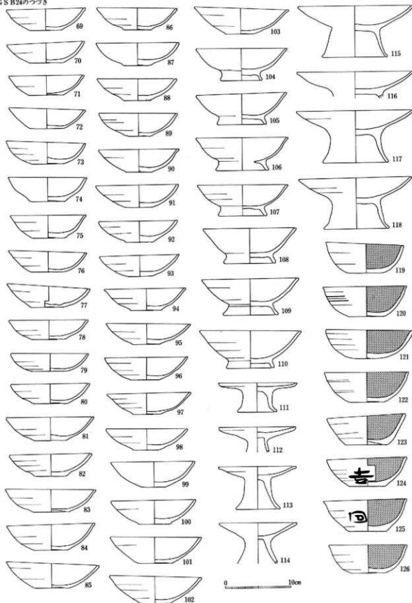
119図 GS B24出土土器実測図(1:4)
