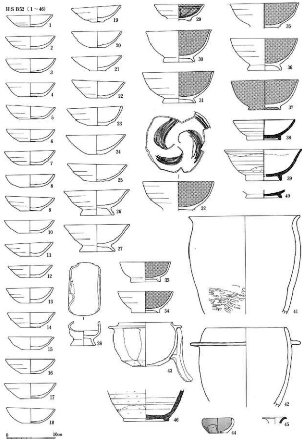
135图 HS B52出土土器实测图(1:4)
