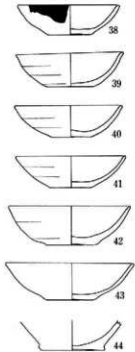
136图 HS B53~55出土土器实测图 (1:4)
