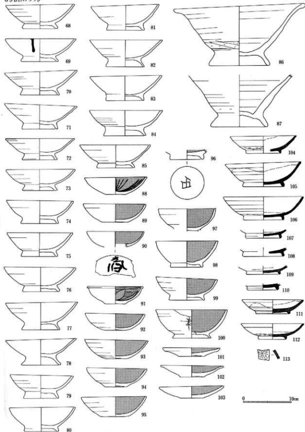
116図 GSB17出土土器実測図(1:4)
