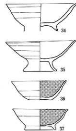
143图 I S B 45·46·51·61出土土器实测图(1:4)
