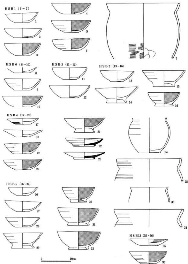
146图 HSB 1 ~ 6 · 13出土土器实测图 (1 : 4)
