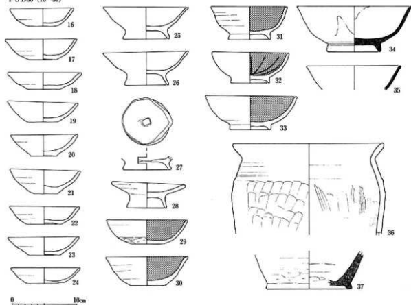
104图 FS B59·60出土土器実測图(1:4)
