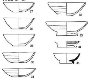
142图 I S B 33·37·75·76出土土器实测图(1:4)
