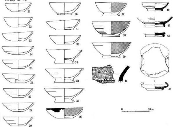
122图 GSB26·32出土土器实测图(1:4)
