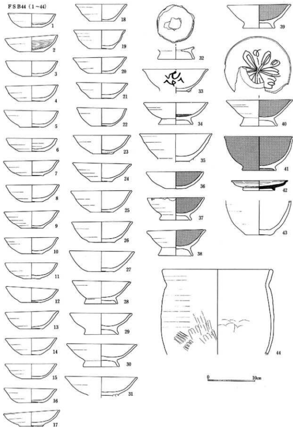
95图 FSB44出土土器实测图(1:4)
