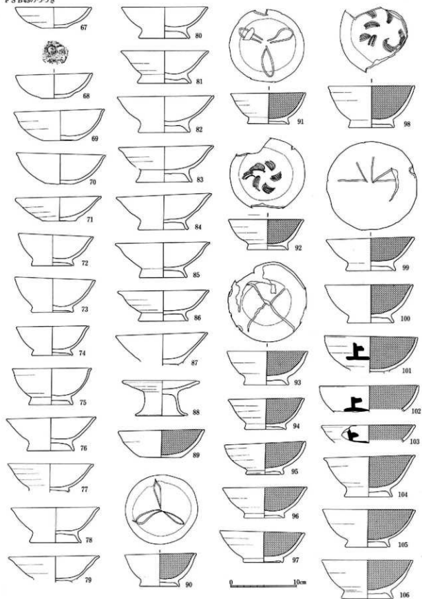
97図 FSB45出土土器実測図(1:4)
