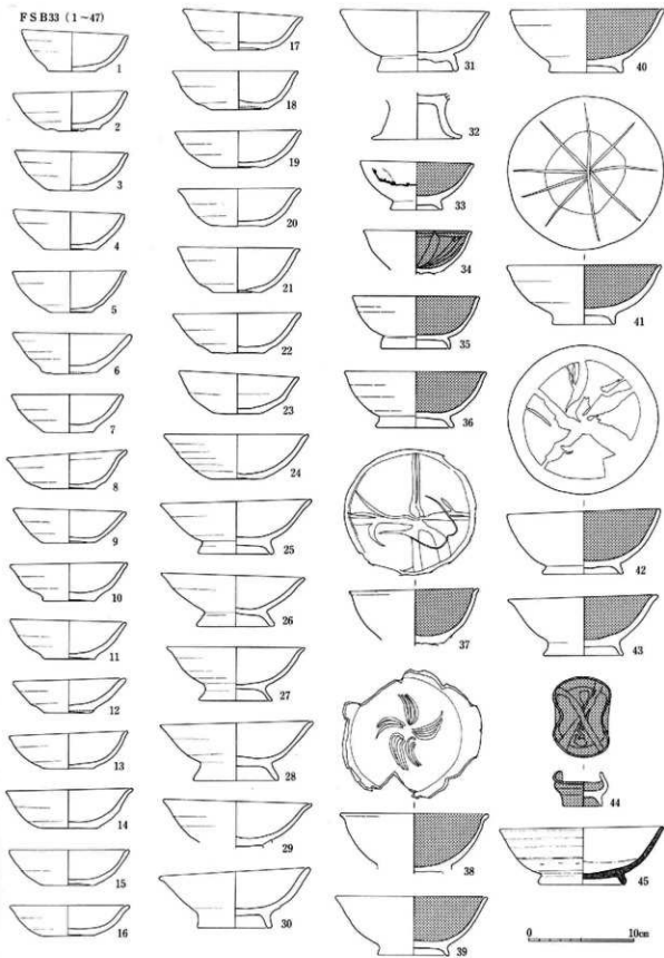
90图 FS B33出土土器实测图 (1:4)
