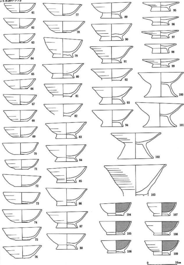
126図 GSB28出土土器実測図(1:4)
