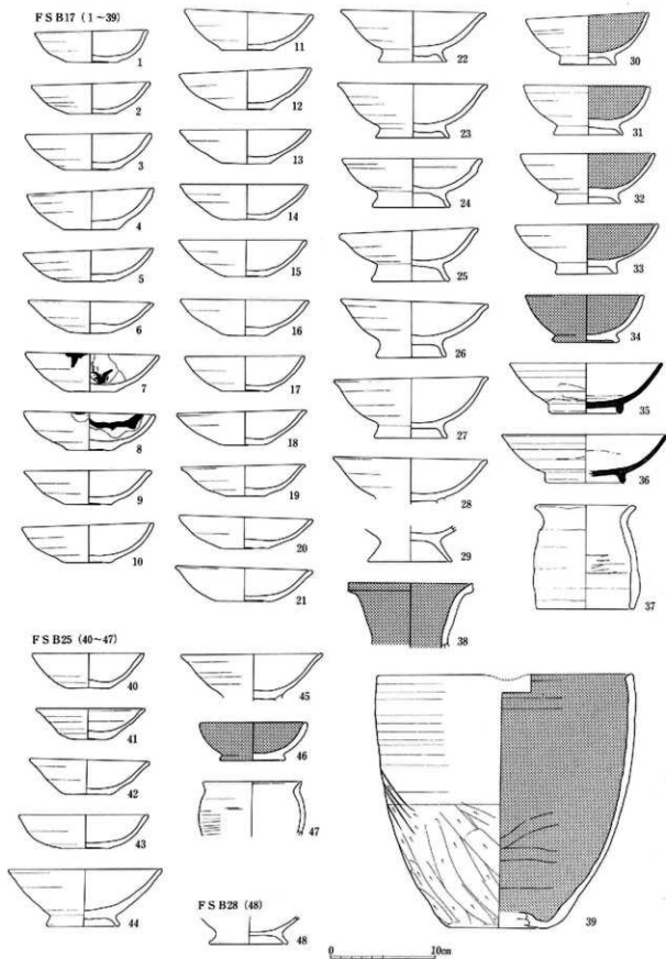
87图 FS B17·25·28出土土器实测图(1:4)
