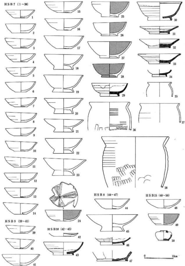
147图 HSB 7~9·15·18出土土器实测图(1:4)
