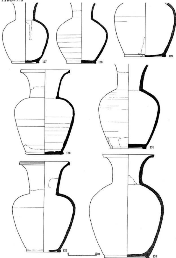
99図 FS B45出土土器実測図 (1 : 4)
