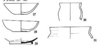
100図 FSB45~47・51出土土器実測図(1:4)
