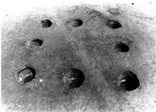
F-10号掘立柱建物址
