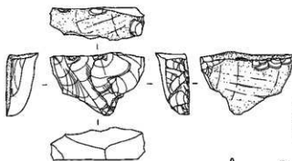
第3地点 石器実測図 68 (石核 18) (貫ノ木遺跡)
