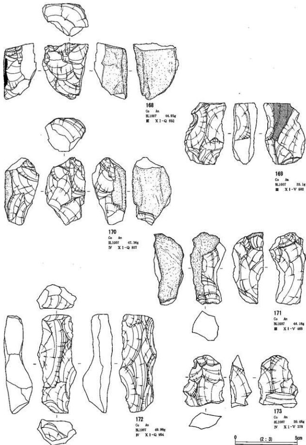
第1地点 石器実測図 29 (石核 1) (貫ノ木遺跡)
