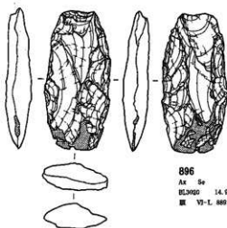
第3地点 石器実測図 23 (槍先形尖頭器 2・斧形石器 1) (貫ノ木遺跡)
