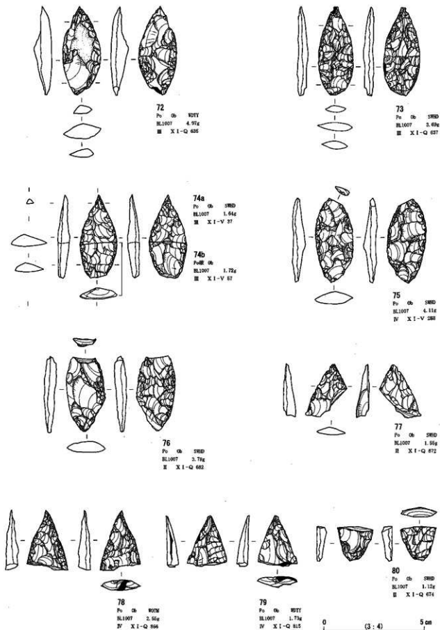
第1地点 石器実測図9(槍先形尖頭器1)(貫ノ木遺跡)
