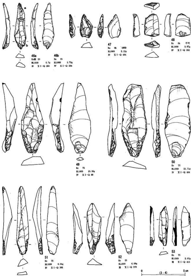
第1地点 石器実測図6 (ナイフ形石器6) (貫ノ木遺跡)
