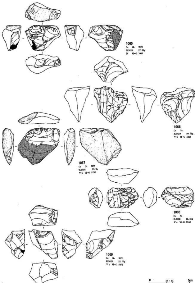
第3地点 石器実測図66(石核16)(貫ノ木遺跡)
