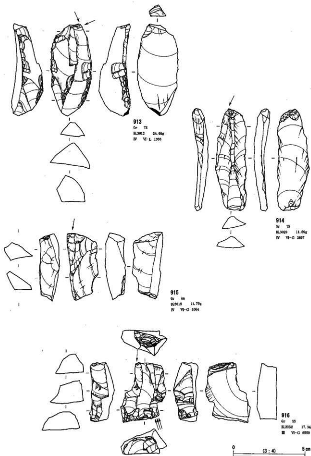
第3地点 石器実測図 32 (影器 2) (貫ノ木遺跡)
