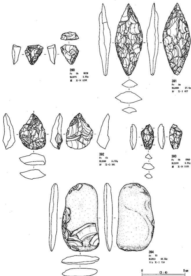
第2地点 石器実測図 25 (槍先形尖頭器5・斧形石器1) (貫ノ木遺跡)
