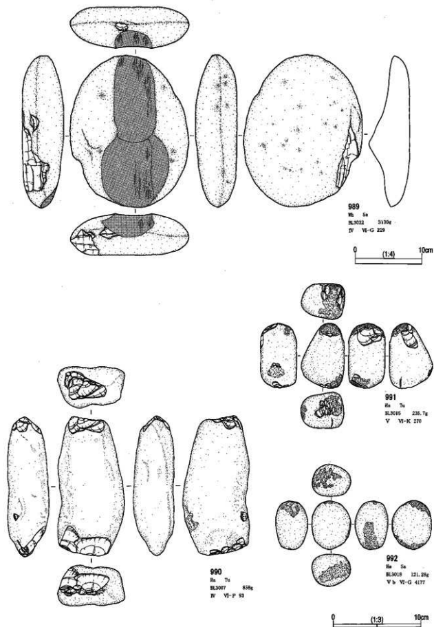
第3地点 石器実測図 49 (礫石3・敲石1) (頁ノ木遺跡)
