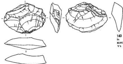
第1地点 石器実測図 24 (攪器 9・攪器状石器) (貫ノ木遺跡)
