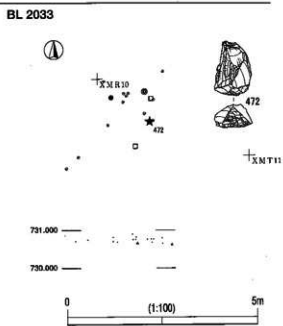
第 2 地点 BL2031・2032・2033 遺物分布図 (貫ノ木遺跡)
