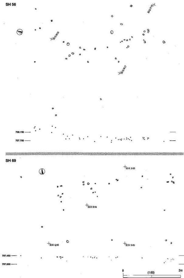
第1地点 SH 56・69 遺物分布図 (貫ノ木遺跡)
