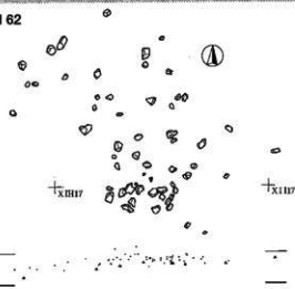
第2地点 SH 61・62・66・67 遺物分布図 (頁ノ木遺跡)
