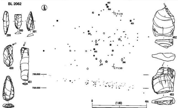
第2地点 BL2061・2062 遺物分布図 (貫ノ木遺跡)
