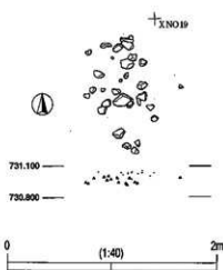
第2地点 SH 154・156・157・158・159・160 遺物分布図 (貫ノ木遺跡)
