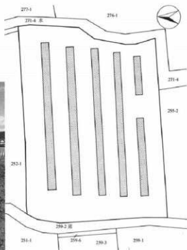
向畑調査全体図 (1:500)
