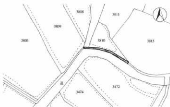
内山中村遺跡調査全体図（1：1,000）
