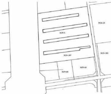
中原遺跡群 20 調査全体図 (1:1,000)
