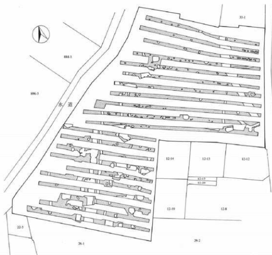
香屋前道路群調査全体図 (1:1,000)
