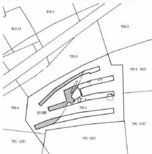
芝宮遺跡群 11 調査全体図 (1:1,000)
