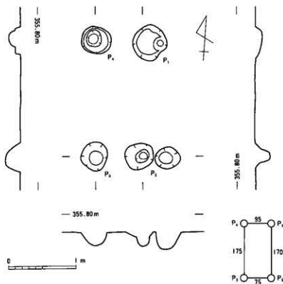
第3図 1号掘立柱建物跡
