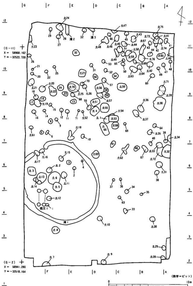
第2図 屋代清水遺跡全体図 (1 : 150)
