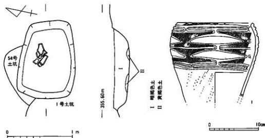
第20図 53号土坑及び出土遺物
