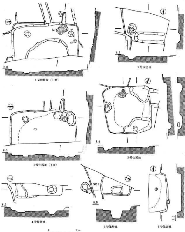
图74 F区住居址实测图(1)
