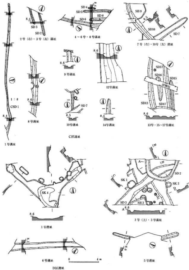
图120 C区·D区沟址、土壤灾测图
