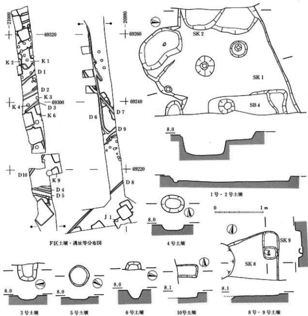
图114 F区土坑实测图
