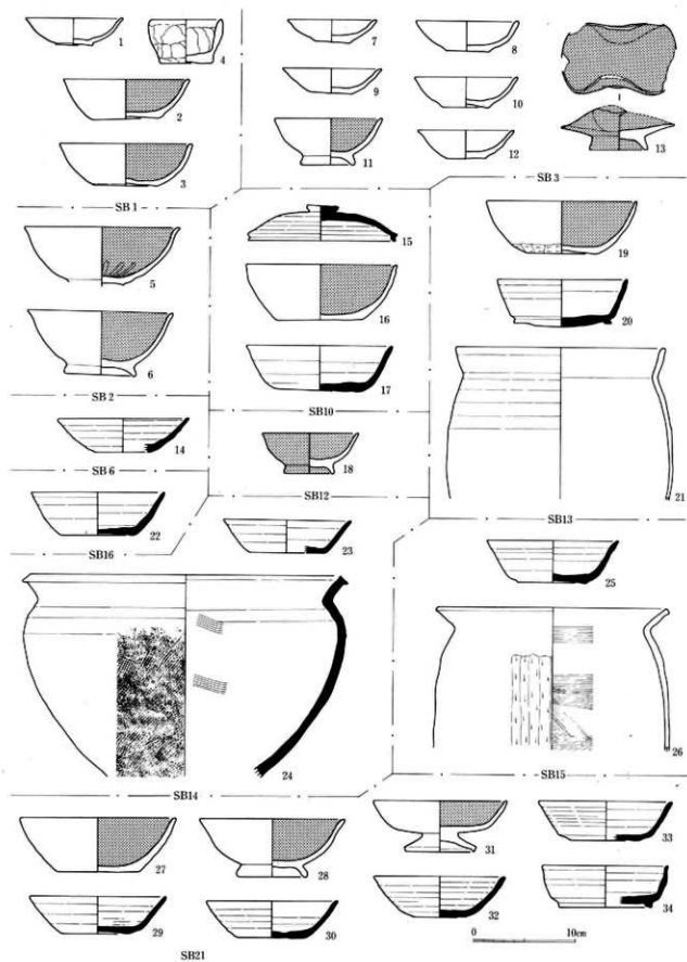
图143 Y区住居址出土土器实测图
