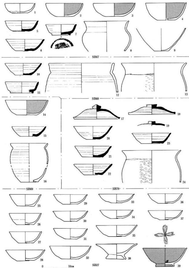
图148 Y区住居址出土土器实测图
