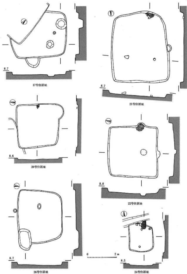
图89 X区住居址实测图(4)
