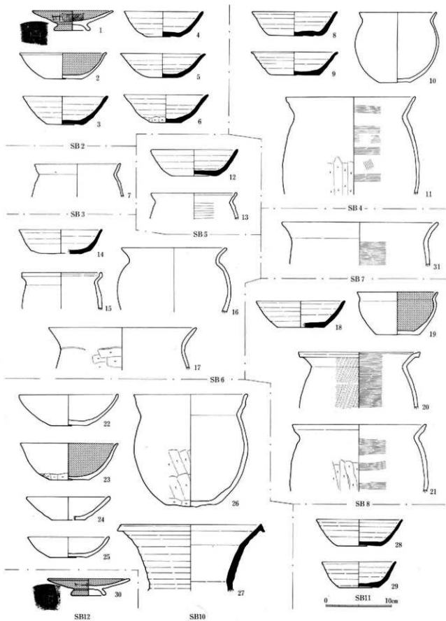
图134 G区住居址出土土器实测图
