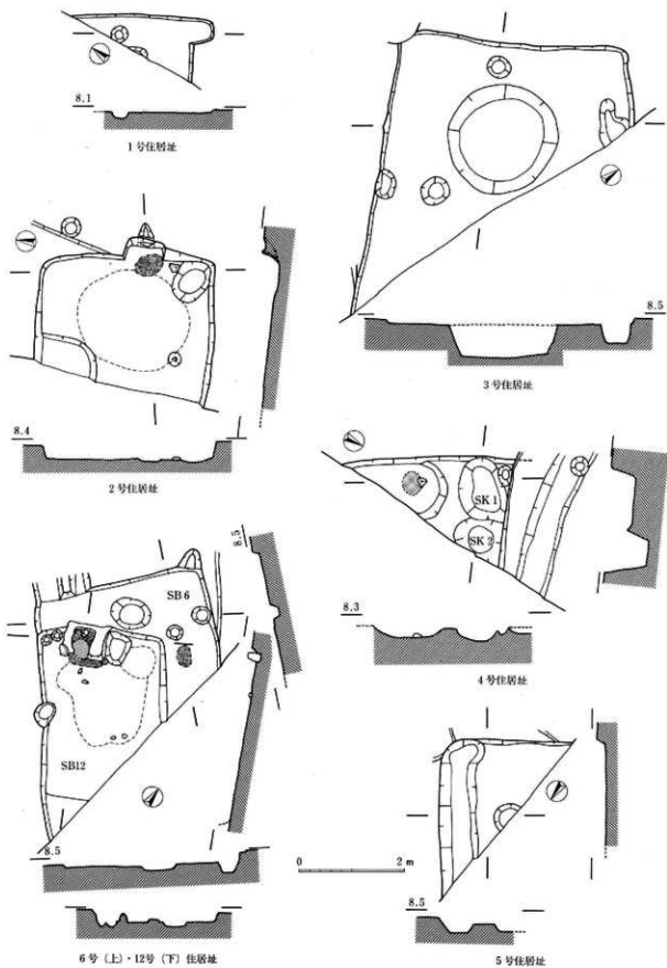
图77 G区住居址实测图(1)
