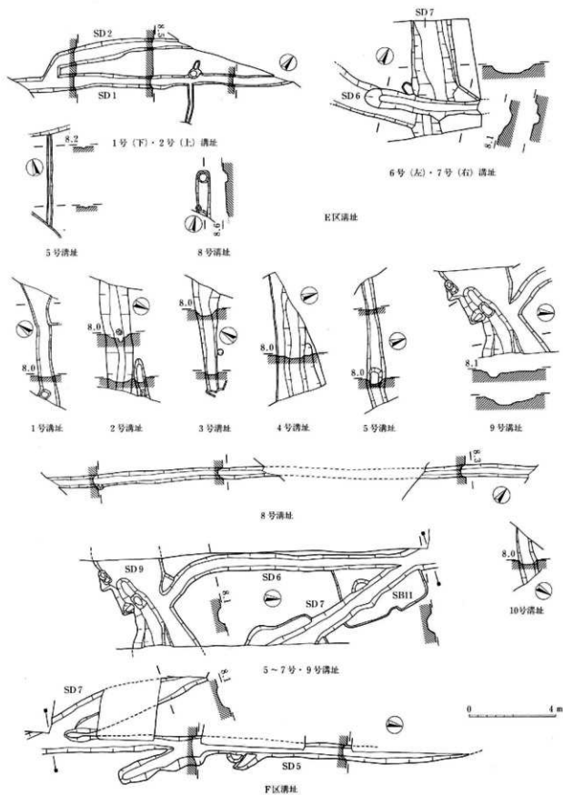
图121 E区·F区清址实测图
