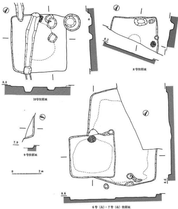
图72 D区住居址实测图(2)
