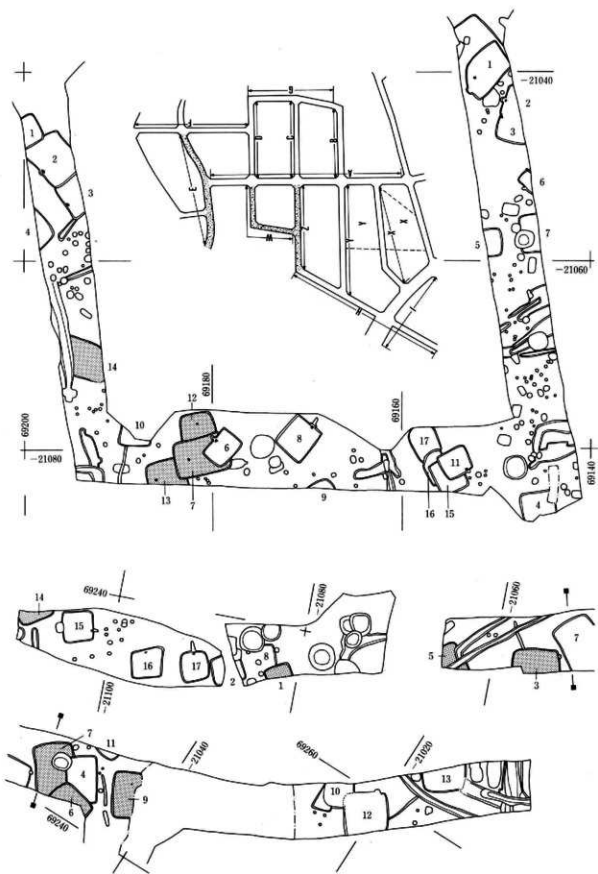
图79 W区・Z区(上)・E区(下)住居址分布图(アミ部弥生时代)
