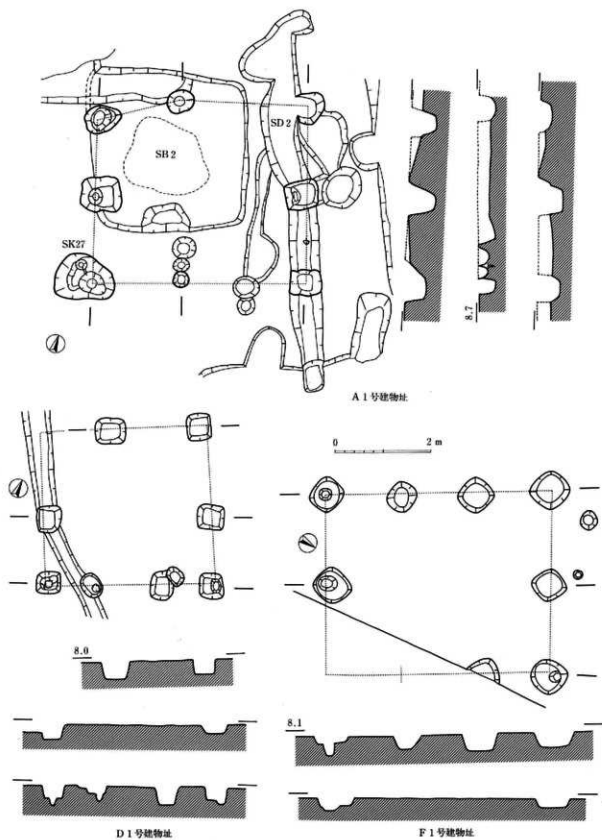
图102 A区·D区·F区建筑物址实测图
