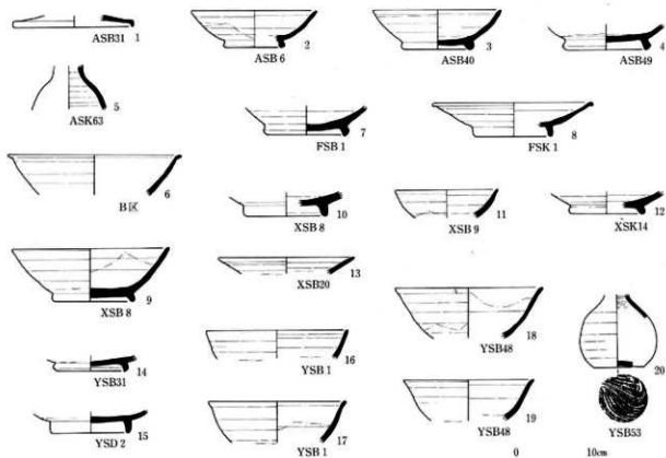
图150 調査地出土灰釉陶器実測図（6～8・20は再掲図）
