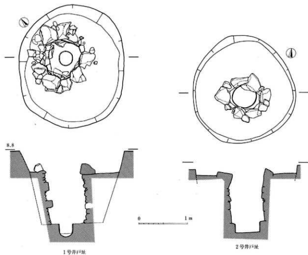
图106 X区井戸址実測図(1:40)
