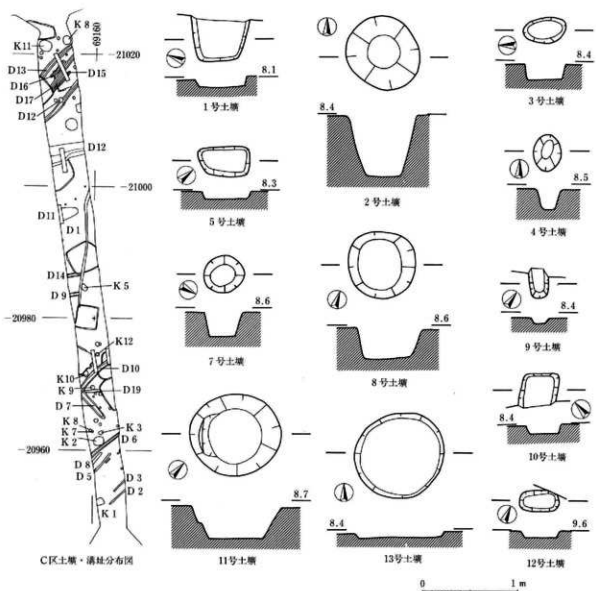
图111 C区土壤实测图
