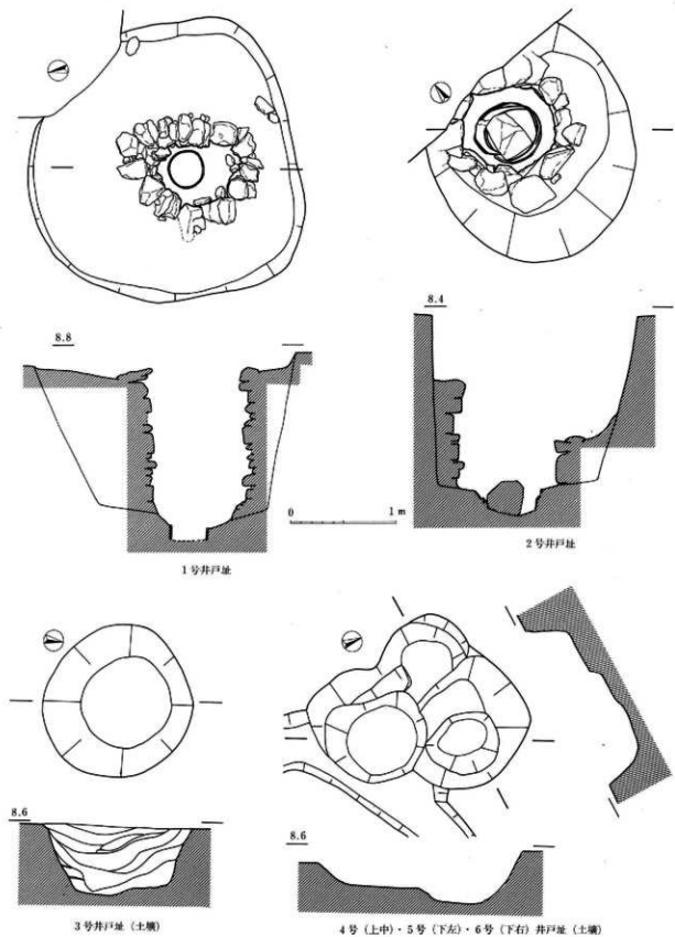
图105 E区井尸址(土壤)实测图(1:40)
