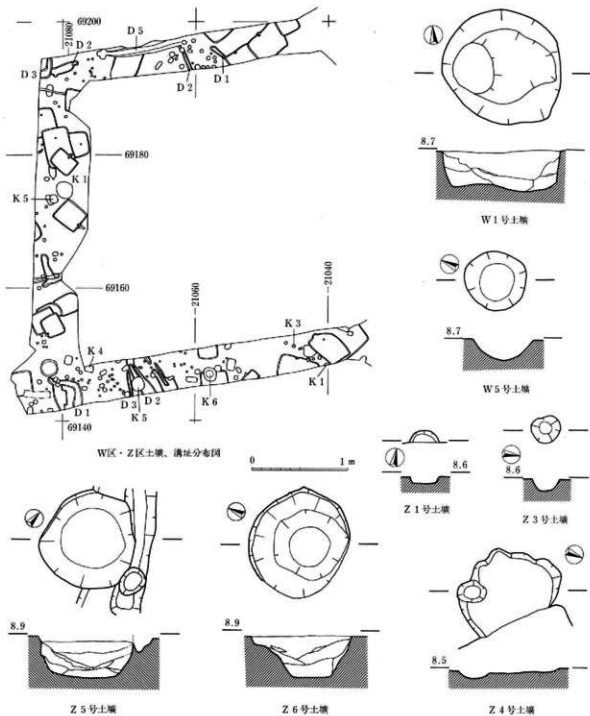
图116 W区・Z区土壤实测图
