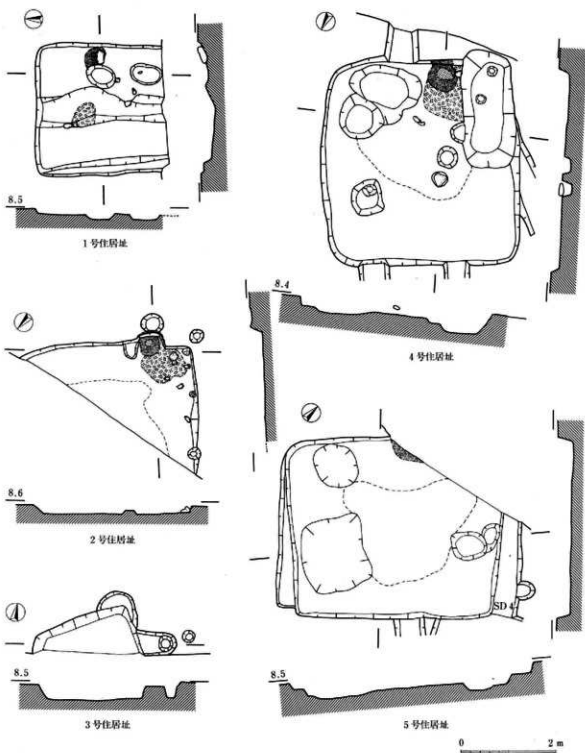
图71 D区住居址实测图(1)
