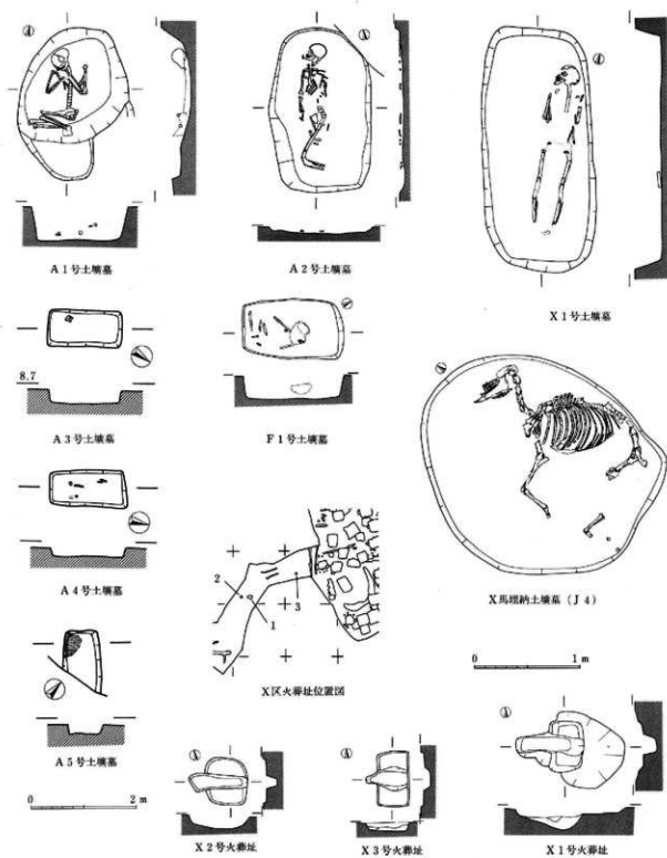
图107 土塚墓·火葬址实测图 (A 3号~5号土塚墓 1:80, 他は 1:40)
