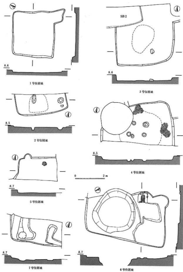
图86 X区住居址实测图(I)
