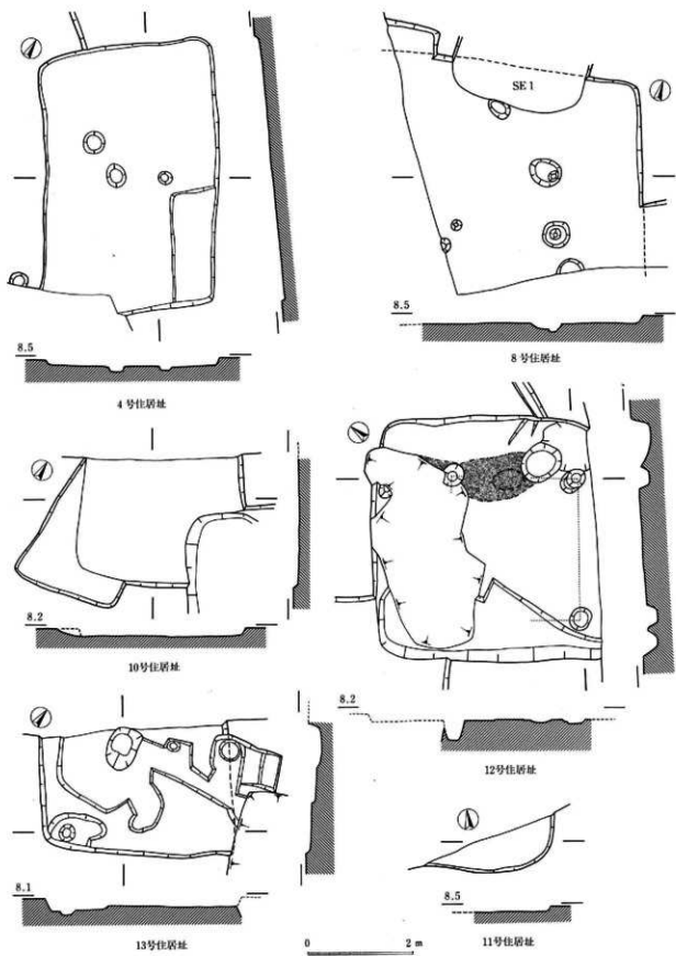
图80 E区住居址实测图(1)
