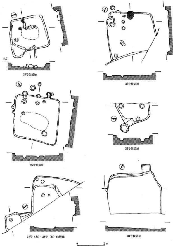
图64 A区住居址实测图(4)
