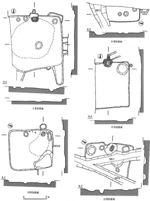
图75 F区住居址实测图(2)
