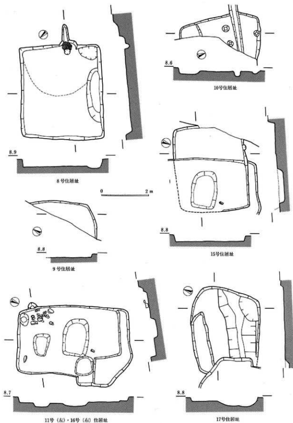
图83 W区住居址实测图(2)
