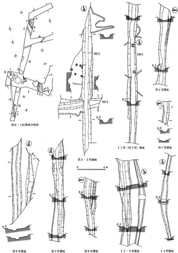
图122 H区·I区沟址实测图
