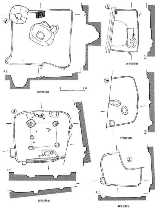
图90 X区住居址实测图(5)
