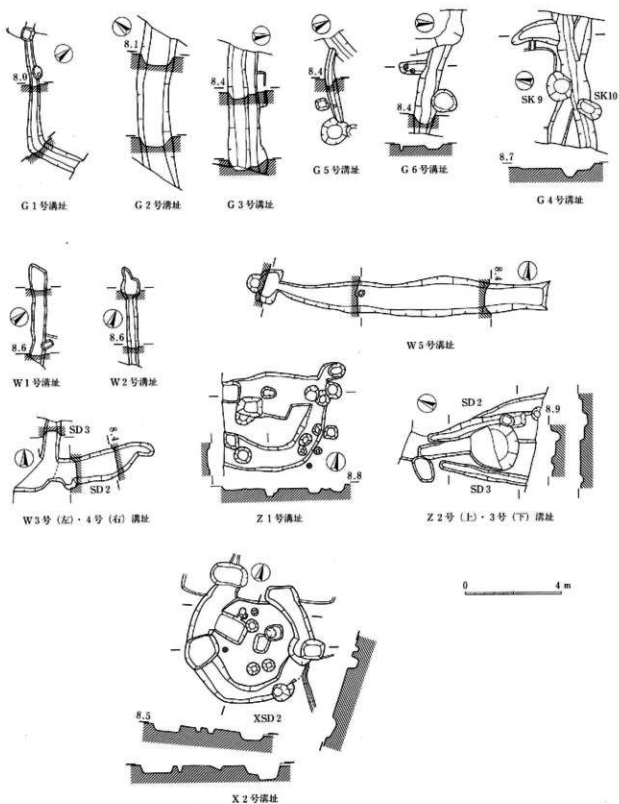
图123 G区·W区·Z区·X区清址实测图
