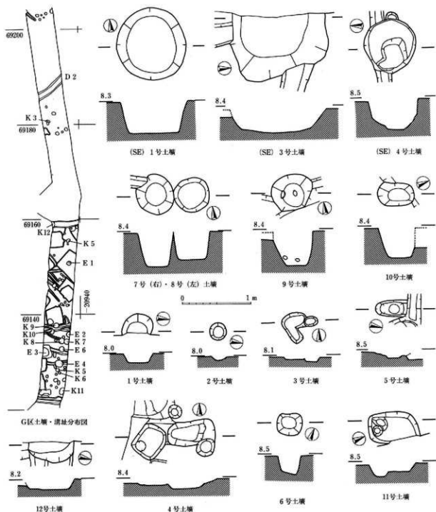
图115 G区土壤实测图
