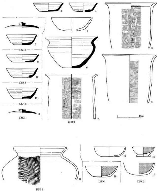
图129 C区·D区住居址、土塚、溝址出土土器実測図
