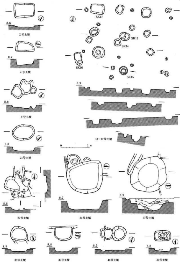
图118 X区·Y区土坑实测图
