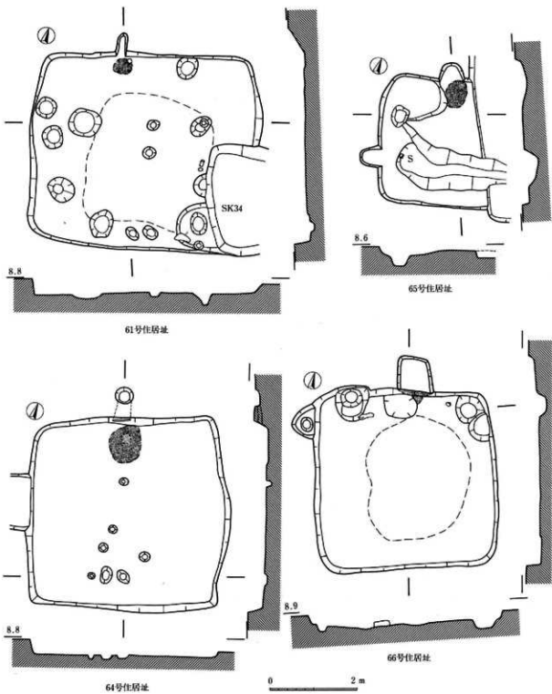
图100 Y区住居址实测图(8)
