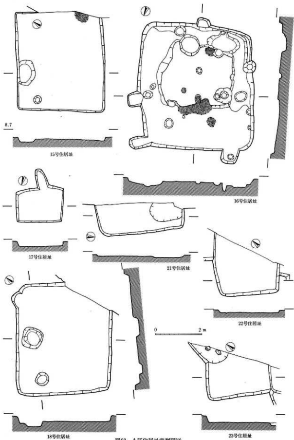
图63 A区住居址实测图(3)
