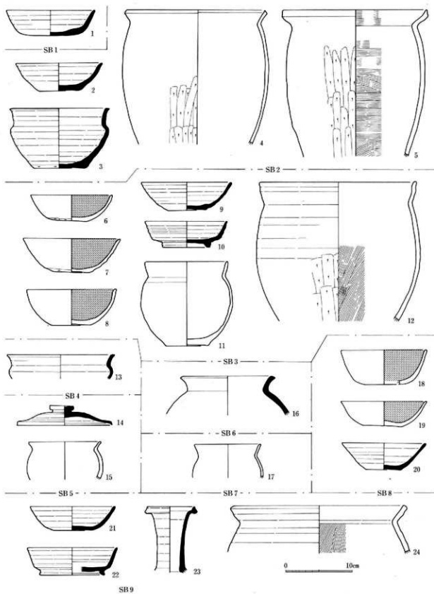
图127 B区住居址出土土器实测图
