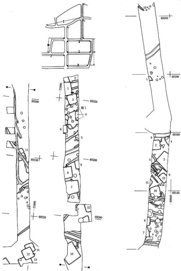
图73 F区(左)·G区(右)住居址分布图
