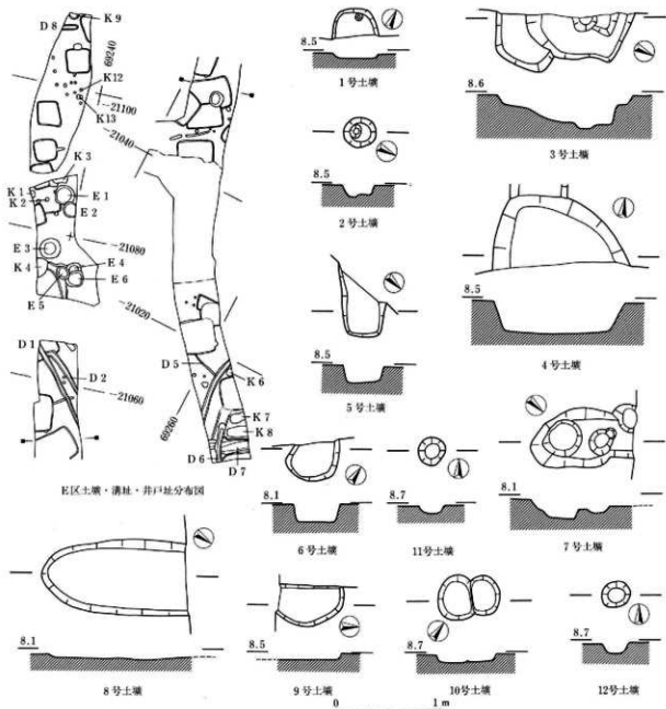
圖113 E区土坑実測図
