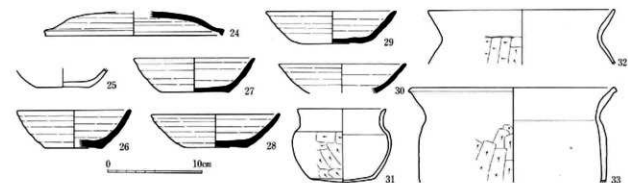
图137 X区住居址出土土器实测图
