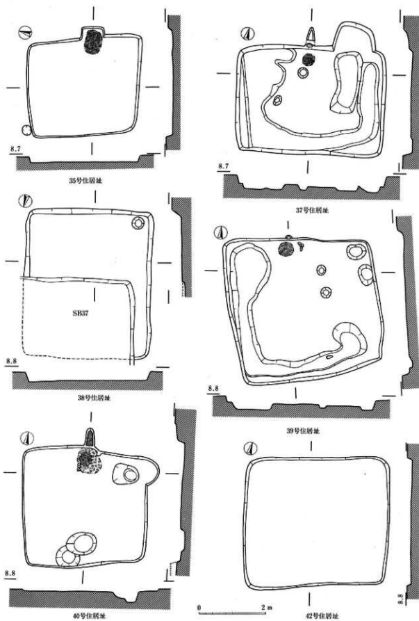
图91 X区住居址实测图(6)
