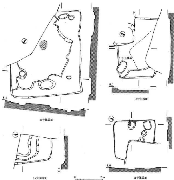
图76 F区住居址实测图(3)
