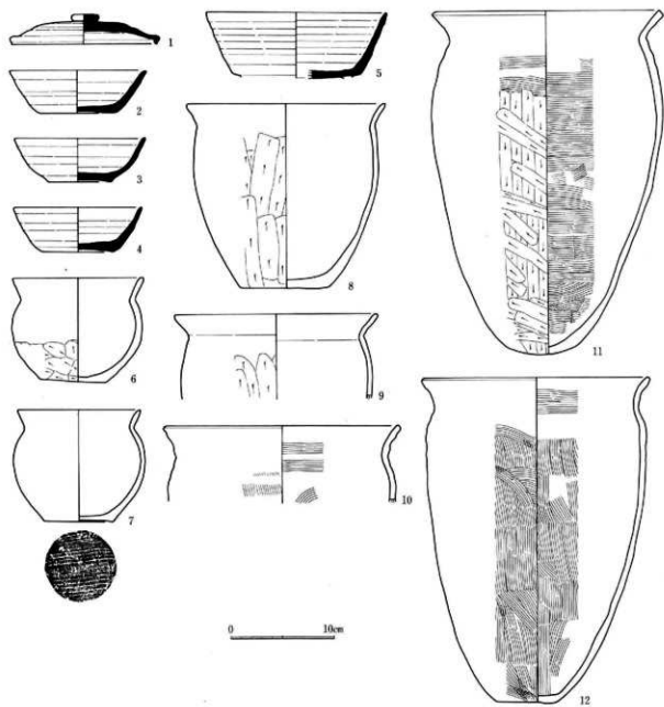
图138 X区19号住居址出土器实测图
