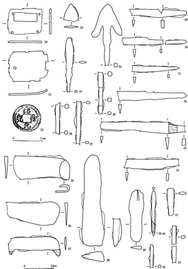
图152 金属製品実測図 (20~22 1:1、他は1:2)
