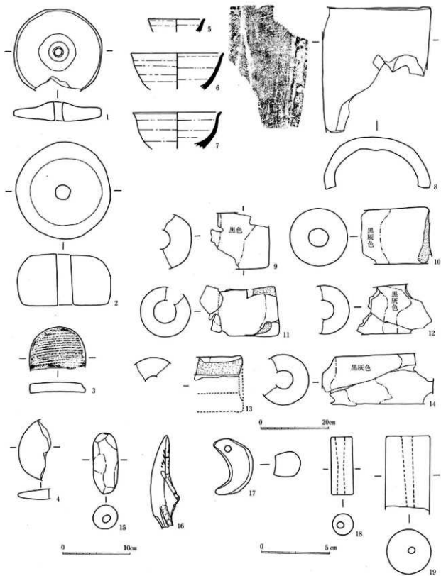
图151 土製品・角製品・石製品実測図 (5~14 1:4、17~19 1:1、他は1:2)
