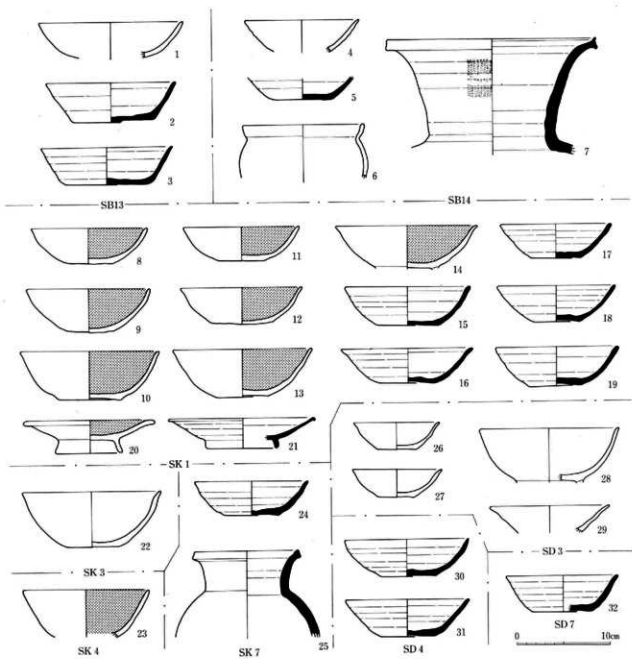
图133 F区住居址、土坑、溝址出土土器实测图
