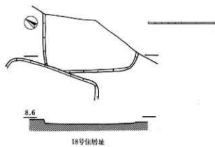
图81 E区住居址实测图(2)
