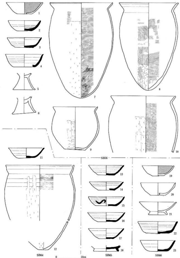
图147 Y区住居址出土土器实测图
