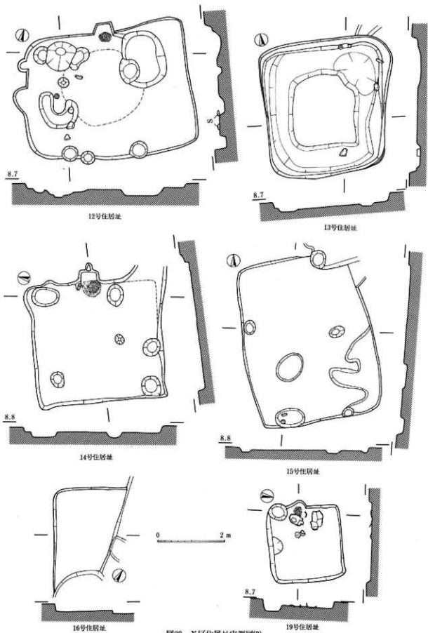
图88 X区住居址实测图(3)
