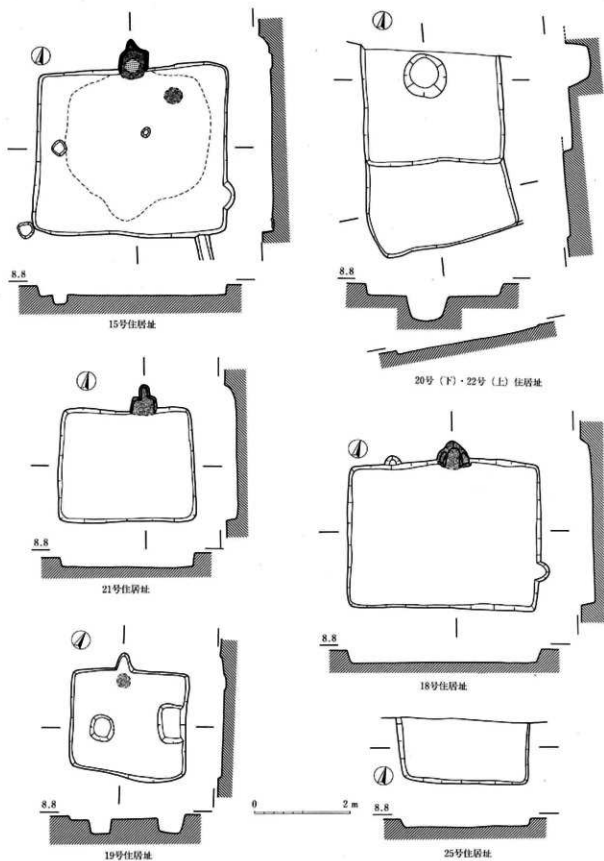
图95 Y区住居址实测图(3)
