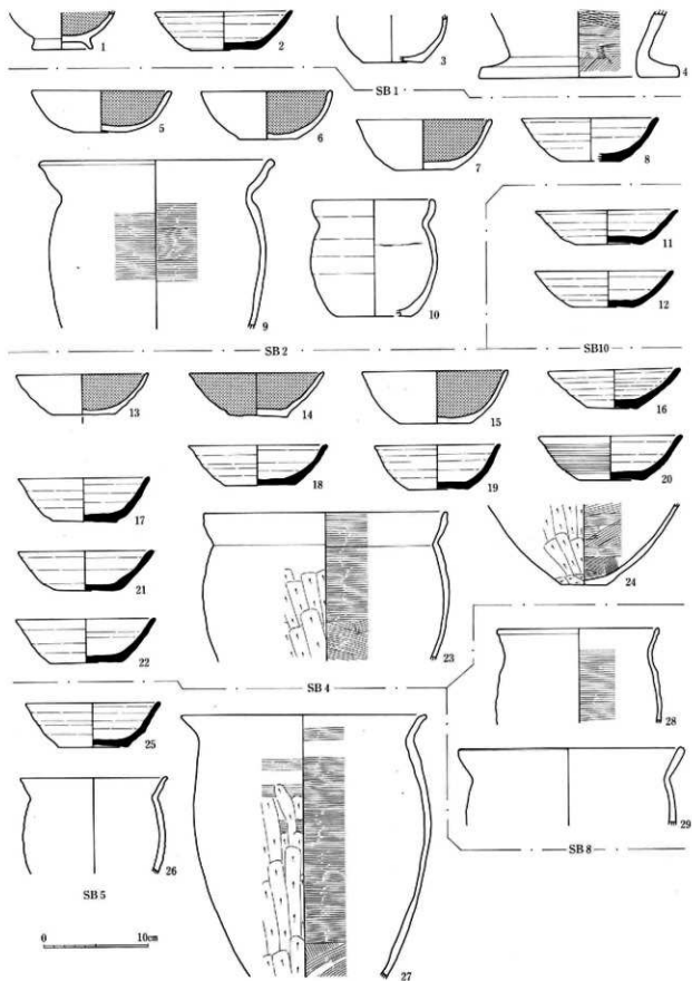
图130 D区住居址出土土器实测图
