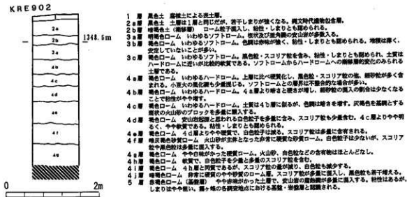
第4図 基本土層堆積図
