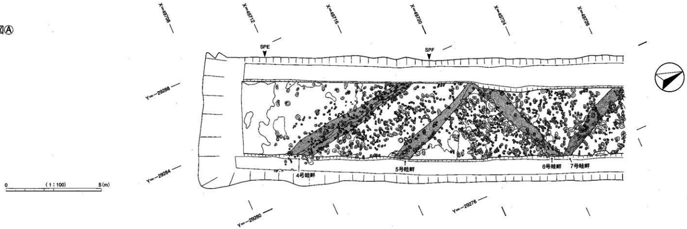
割付図⑤
