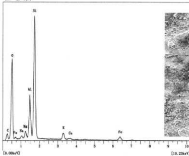
D・E・F. 基部研磨痕のEDX分析チャート
