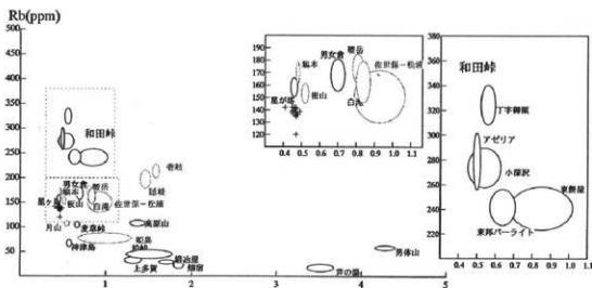
第201図 黒曜石の産地判定図
