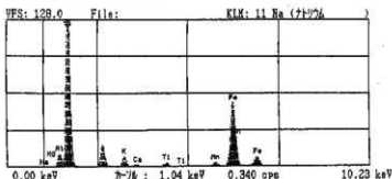
第156図 珪質頁岩Aの鉱物組成
