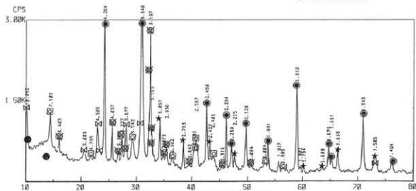
X線回折分析による主な鉱物値
