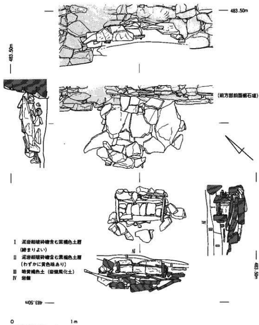
挿図3 第8号組合式箱形石棺
