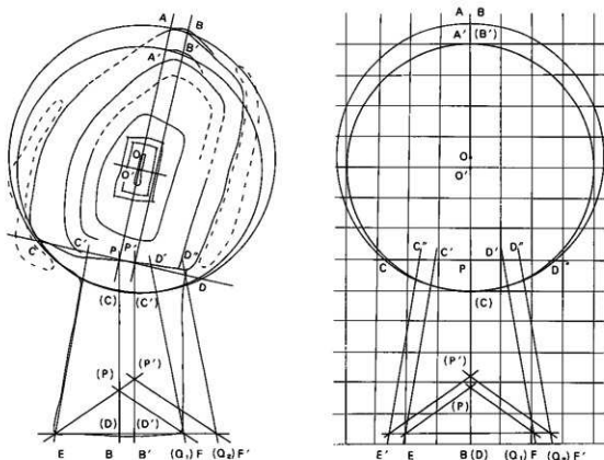
挿図7 森将軍塚古墳の設計企画
