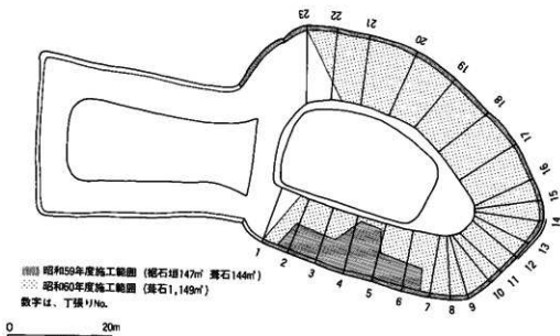
挿図1 昭和60年度復原工事施工範囲
