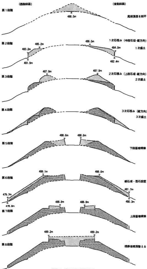
挿図2 後円部墳丘築造過程
