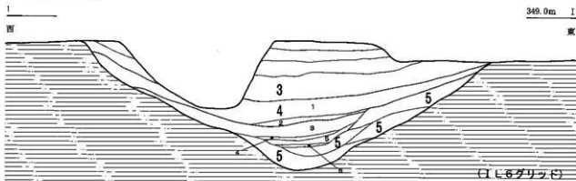
(I'はHグリッド) 【土層断面 I'】 4-1 灰褐色細砂土 土層が最も多く出土する 4-5 灰褐色細砂土 4層よりも灰色がかり強い 4-2 灰褐色細砂土 4-1層より粒子微密、流入層 4層下に炭化粒を含む部分有り (4-4、4-5は同質層) 349.0m J'
