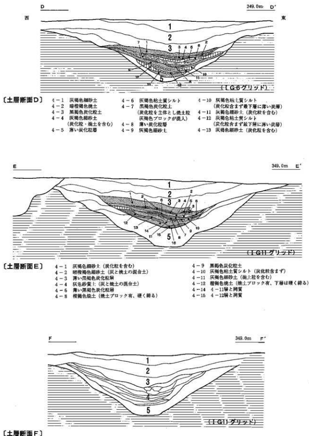
第95図 SD12土層断面D・E・F
