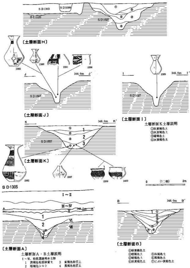
第104図 SD1027・1305土層断面図
