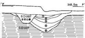
【土層断面F】
