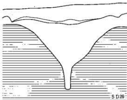
【土層断面B】(II N9 グリッド)
