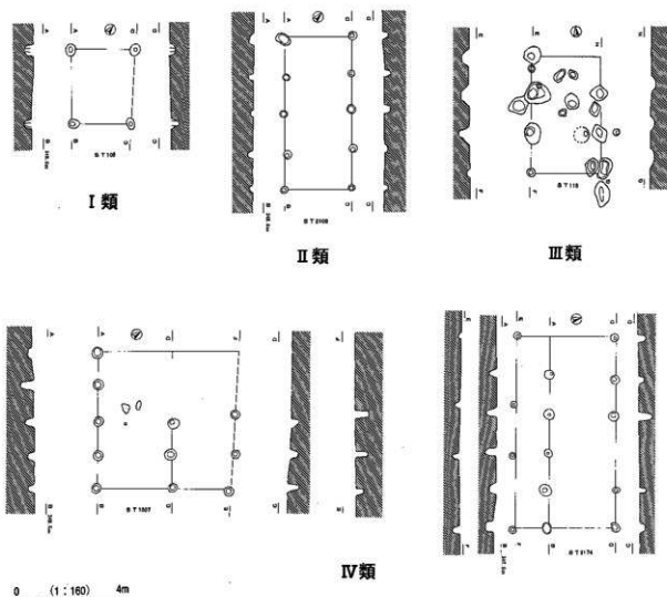
第74図 掘立柱建物址の分類
