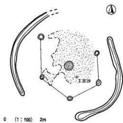
第42図 SBH74
