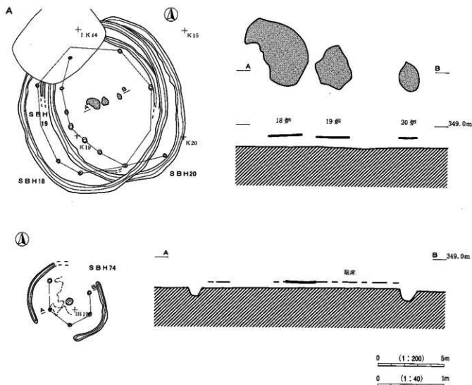
第57図 炉 構造 (1)
