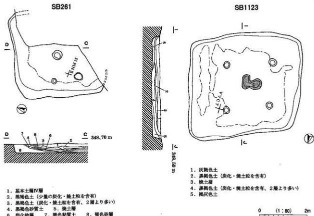
第25図 SB261・1123 実測図
