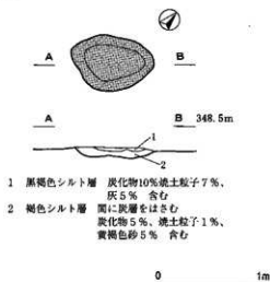
第69図 ST2005炉
