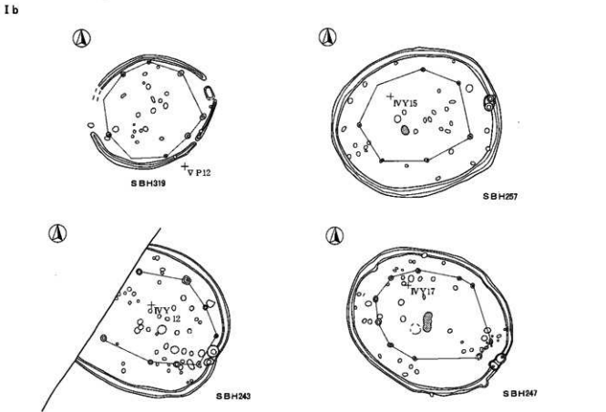
第48圖 柱穴配列 (I)
