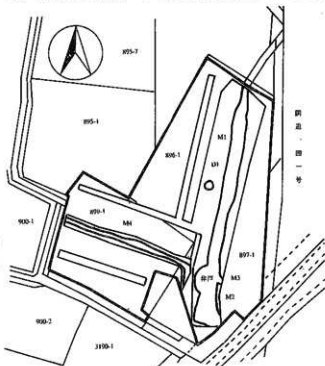
番屋前遺跡群番屋前遺跡Ⅱ調査全体図 (1:1,000)
