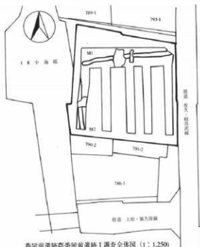
番屋前遺跡群番屋前遺跡 I 調査全体図 (1:1,250)
