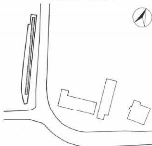
根々井大塚古墳 調査全体図 (1:1,000)
