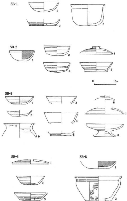
图9 塩崎児童館建設 土器実測图①(1:4)
