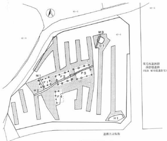
栗毛坂遺跡群 4 A地区検出遺構全体図 (1:500)
