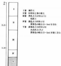
上の原遺跡群1土層柱状図
