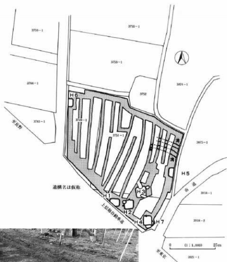
栗毛坂遺跡群11調査全体図 (1:1,000)
