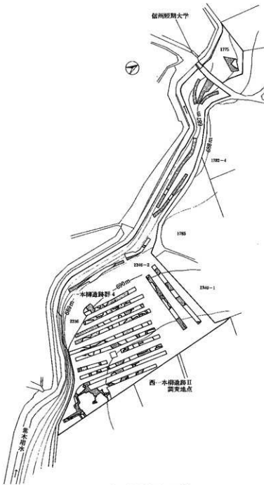
一本柳遺跡群 5 調査全体図 (1 : 1,500)
