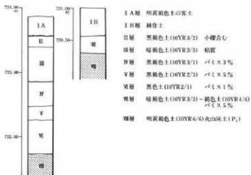
蛇塚A遺跡群1土層柱状図
