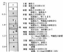
境内遺跡1 土層柱状図
