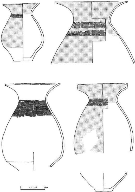
根々井氏館跡 1 トレンチ出土土器実測図 (1 : 4)
