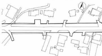
上小平遺跡1調査全体図 (1:1,500)
