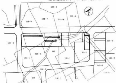
岩村田遺跡群10調査全体図 (1 : 2,000)
