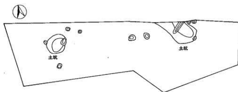
菅田遺跡2検出遺構全体図 (1:80)
