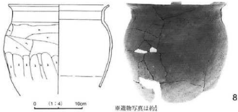
第9図 H2号住居址出土遺物実測図(1)
