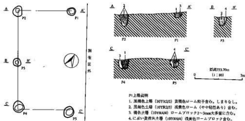
第11図 F1号掘立柱建物址実測図
