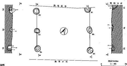
第11図 F1号掘立柱建物址実測図
