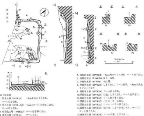
第6図 H2号住居址実測図
