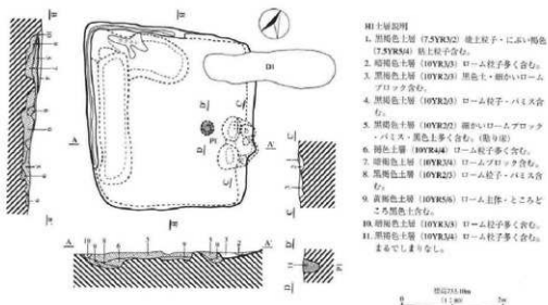
第5図 H1号住居址実測図
