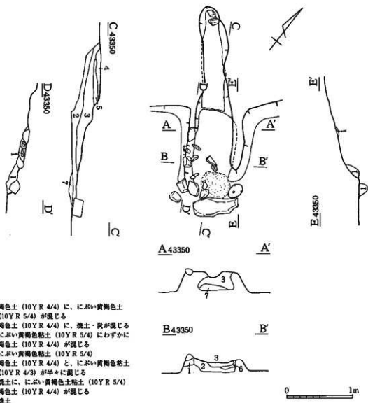
挿図9 SB12カマド
