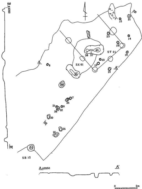
挿圖14 柱穴・穴
