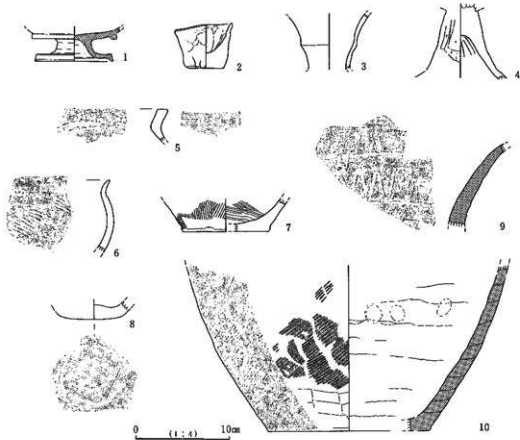
第29図 土坑・溝状遺構出土遺物実測図
