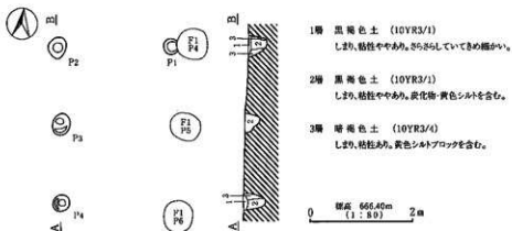
第21図 F2号掘立柱建物址実測図
