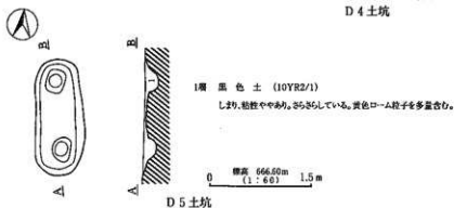
第25図 D 2 . 3 . 4 . 5 号土坑実測図
