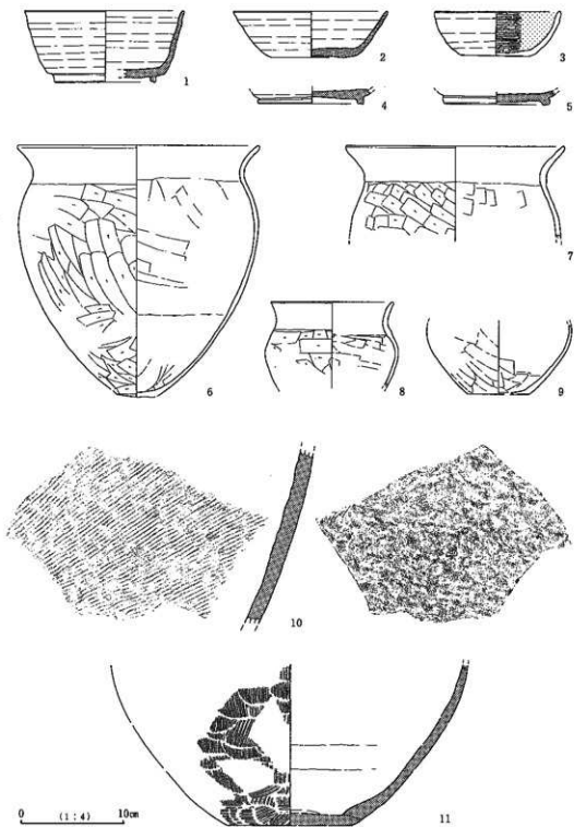
第13图 H3号住居址出土遗物实测图
