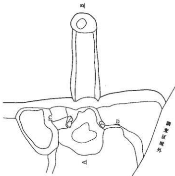
第15図 H4号住居址カマド実測図
