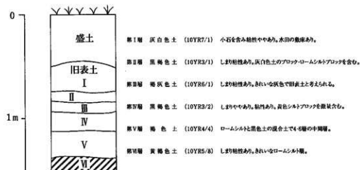
第5図 基本層序模式図
