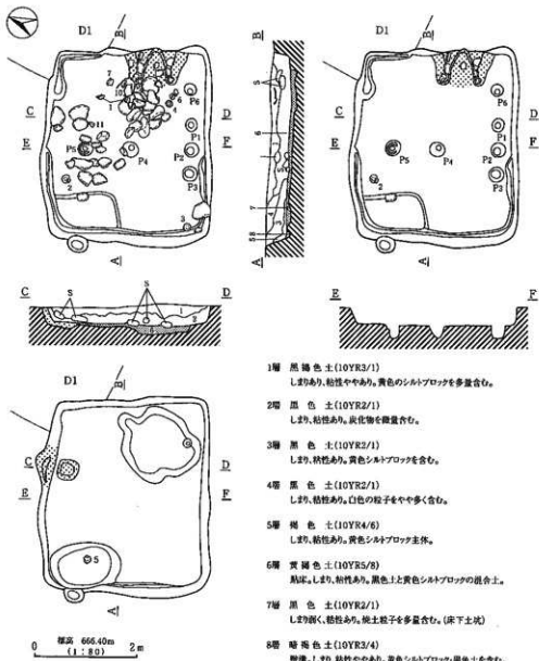
第11図 H3号住居址実測図
