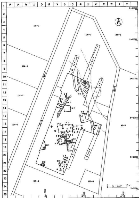
第6図 市道遺跡II調査区全体図
