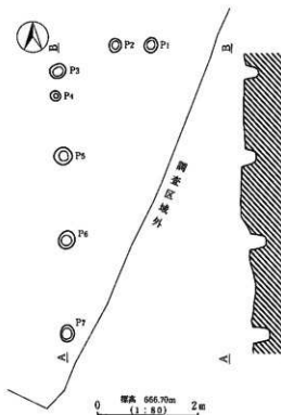
第23図 F4号掘立柱建物址実測図
