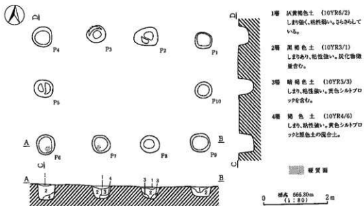
第20図 F1号掘立柱建物址実測図
