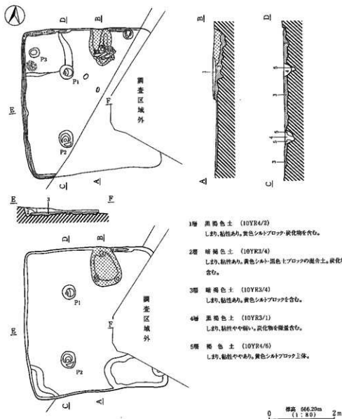
第17図 H5号住居址実測図
