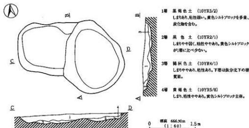
第24図 D1号土坑実測図
