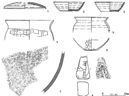
第16図 H4号住居址出土遺物実測図
