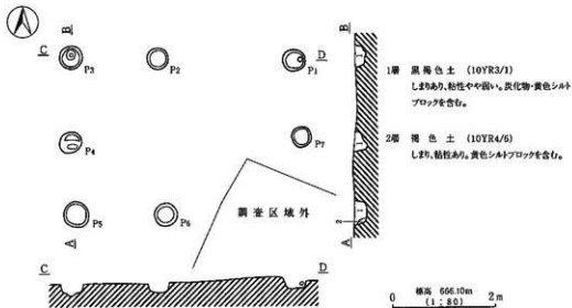
第22図 F3号掘立柱建物址実測図
