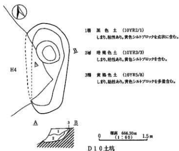
第26図 D 6 . 7 . 8 . 9 . 10号土坑実測図
