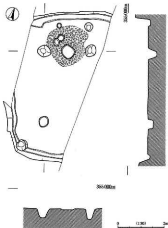
図285 SB154実測図
