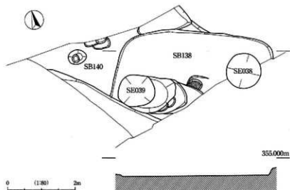
図245 SB138実測図
