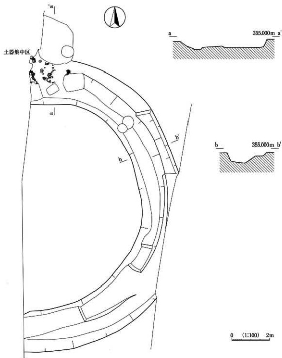
図294 SZ029実測図
