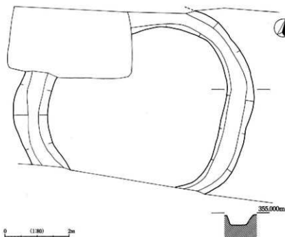
図255 SZ026実測図
