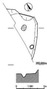
図284 SB159実測図
