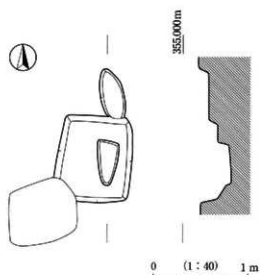
図300 SX025実測図
