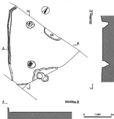
図261 SB147実測図
