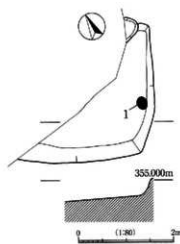
図287 SB158実測図
