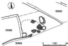
図246 SB134実測図
