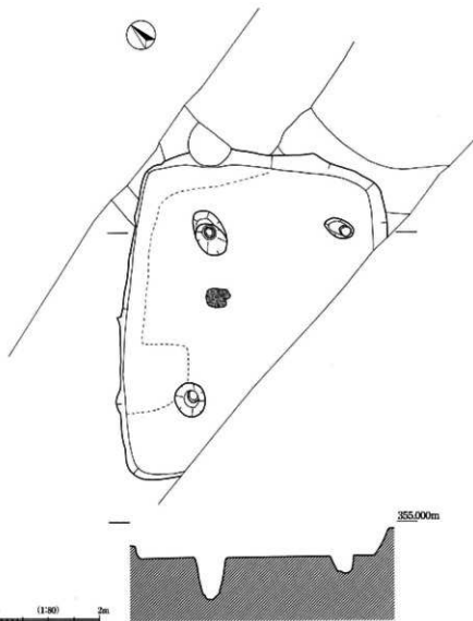
図253 SB144実測図
