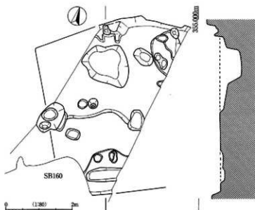
図309 SB165実測図
