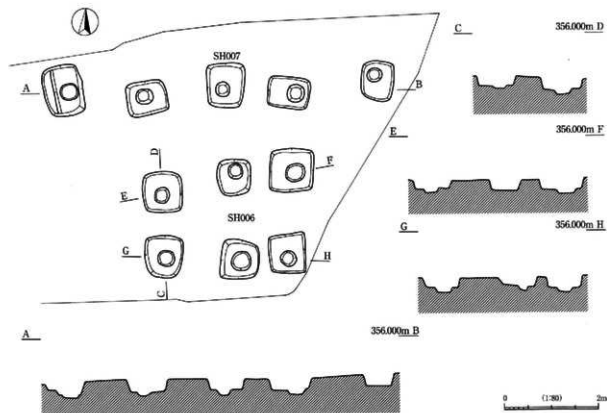
図258 SH006・007実測図
