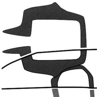
図89 SZ006復元想定図 (S=1/320)
