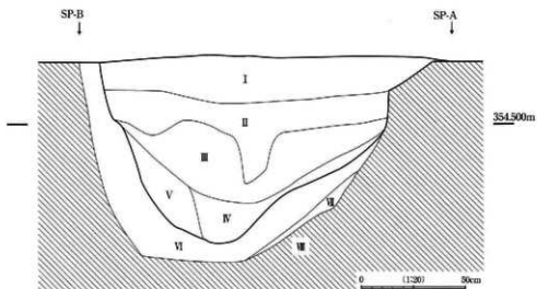
図119 周溝堆積土層実測図 (S=1/20)
