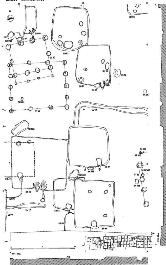
图版28 遗构实测图16
