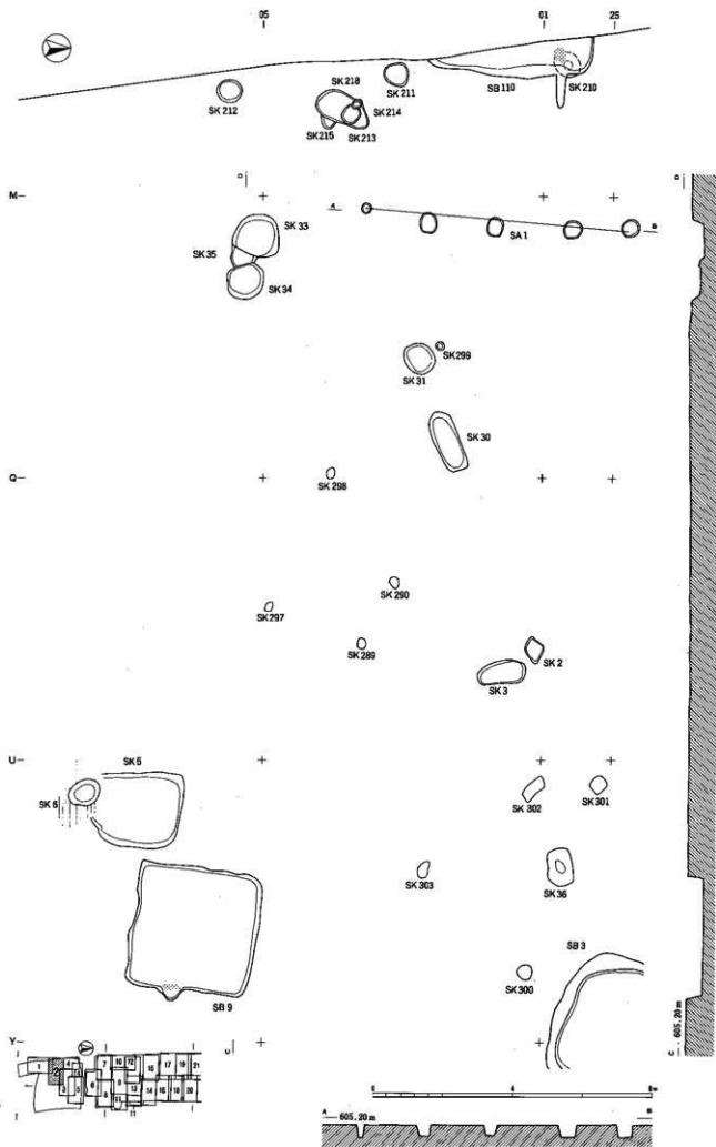
図版14 遺構実測図2
