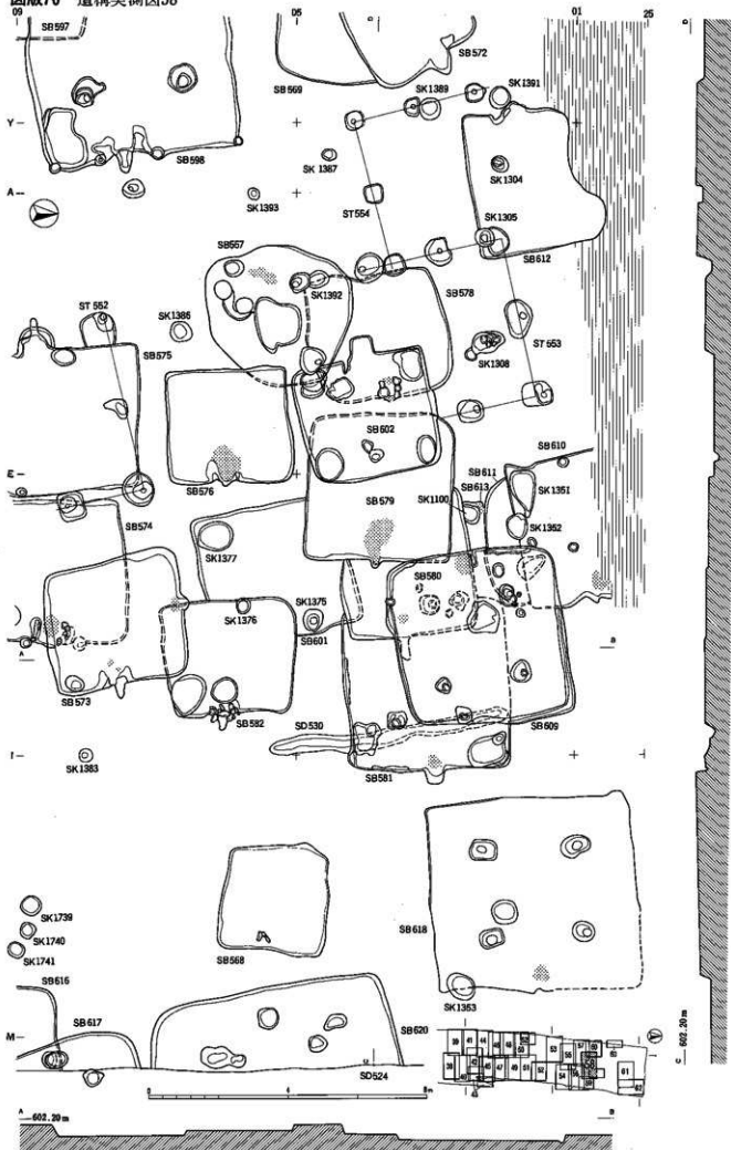
图版70 遺構実測図58
