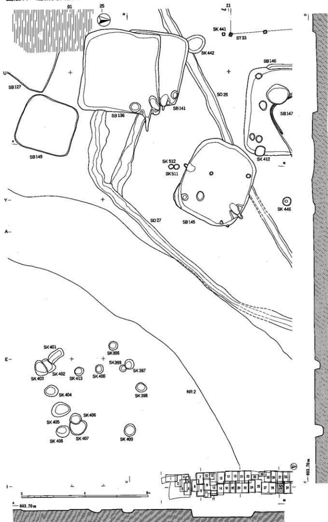
図版44 遺構実測図32
