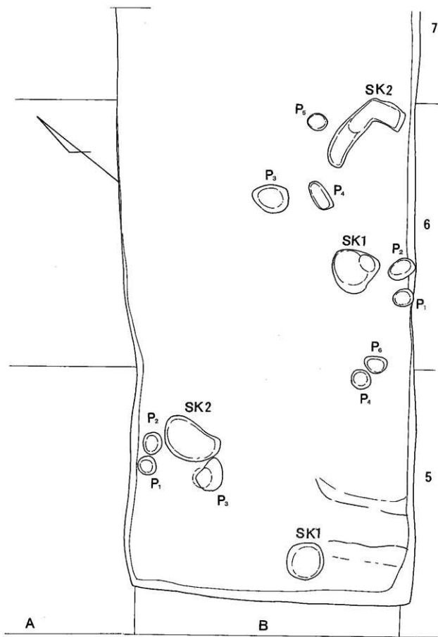
圖5 遺構分布圖2(1:50)
