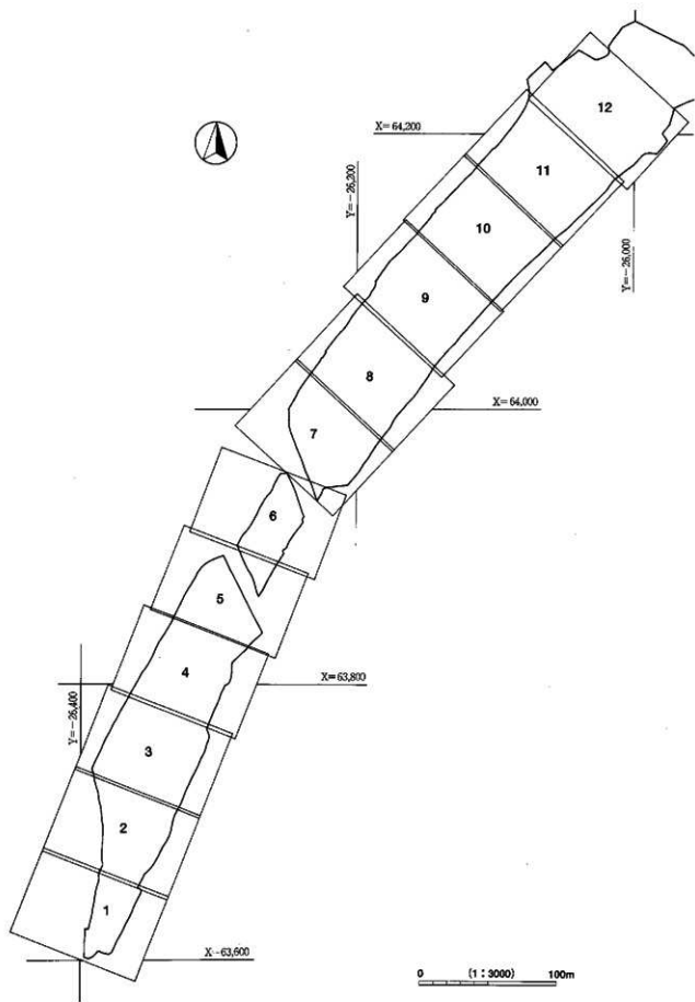
図版 2 遺構配置図割付図
