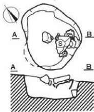
第75図 536P 平・断面図 (1:30)
