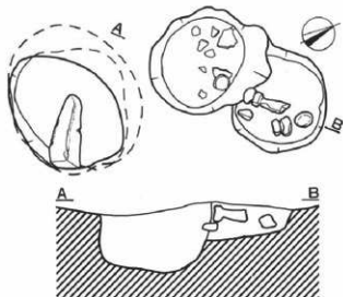
第69図 476P・477P 平・断面図 (1:30)
