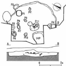
第23図 15号住居跡平面図 (1:80)
