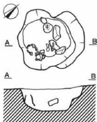
第74図 532P 平・断面図 (1:30)
