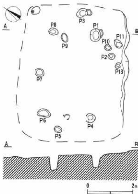
第12図 5号住居跡平面図(1:80)
