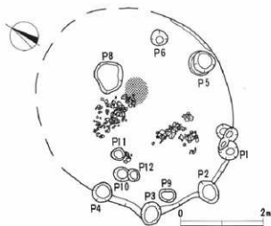
第5図 3号住居跡平面図(1:80)
