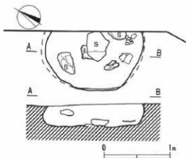
第30図 17P 平・断面図(1:80)
