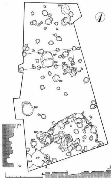
第47図 長塚遺跡遺構全体図 (1:120)
