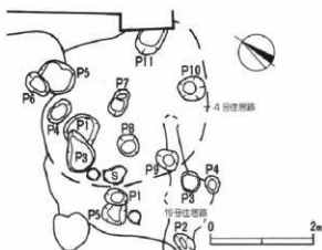
第9図 4・19号住居跡平面図(1:80)
