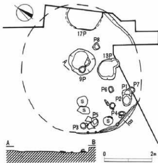
第25図 16号住居跡平面図 (1:80)
