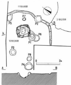
第16図 10号住居跡平面図 (1:80)
