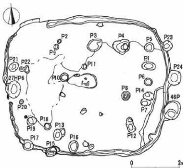
第13図 67号住居跡平面図(1:80)
