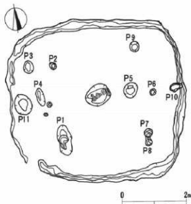
第17図 66号住居跡平面図(1:80)
