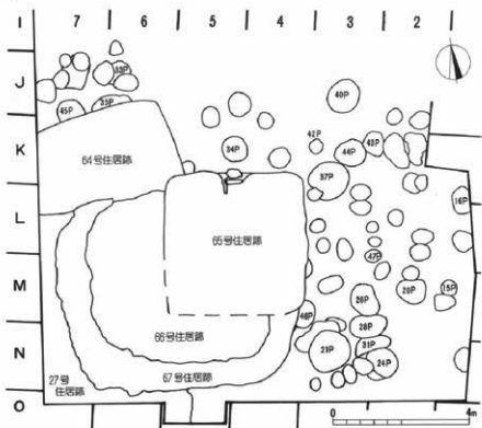
第7図 海戸遺跡遺構配置図(1:120)
