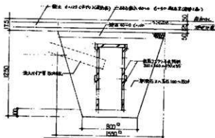
地下埋设排水 止水栓 断面图
