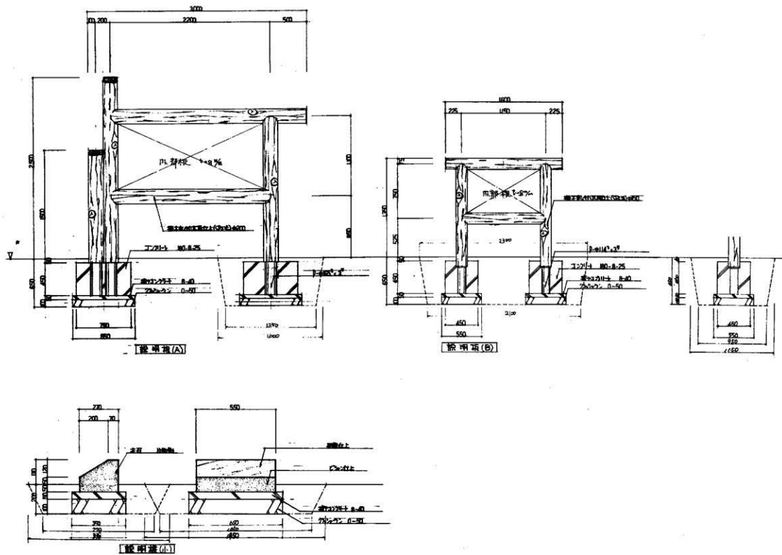
第9区 説明板詳細図
