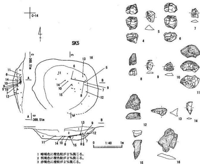
第9図 A地点遺構図(4)
