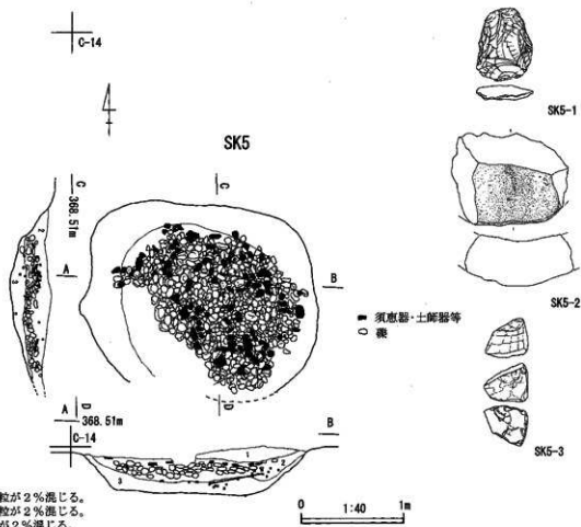
第6図 A地点遺構図(3)
