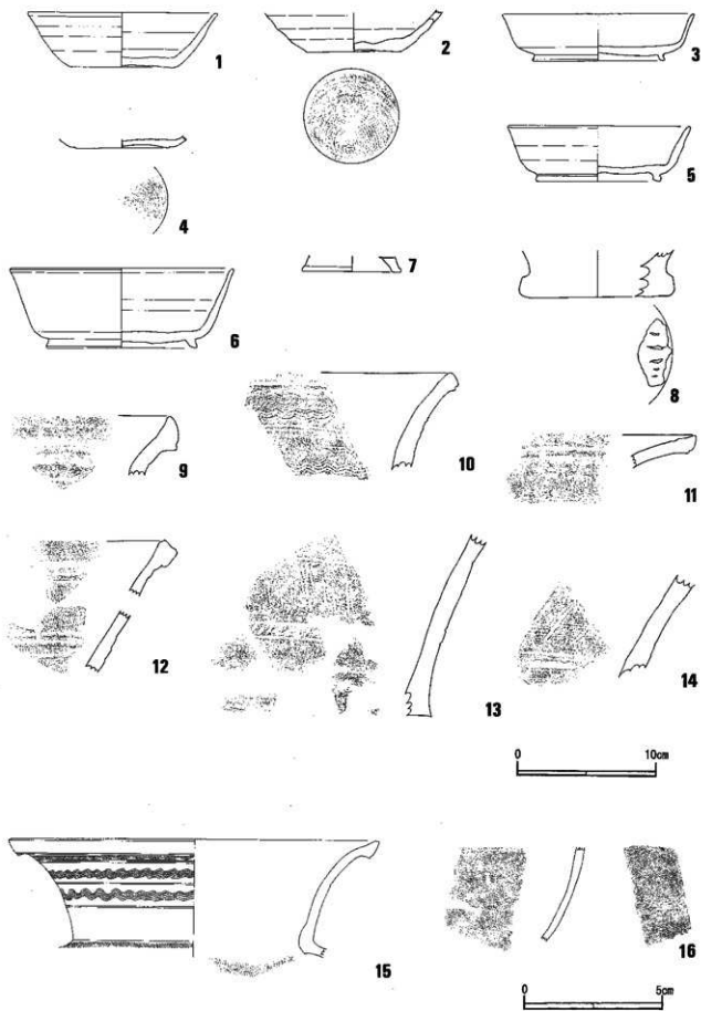
第13图 A地点出土遗物(1)
