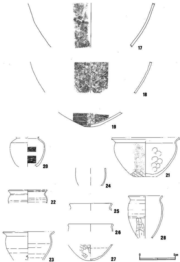
第14图 A地点出土遺物(2)
