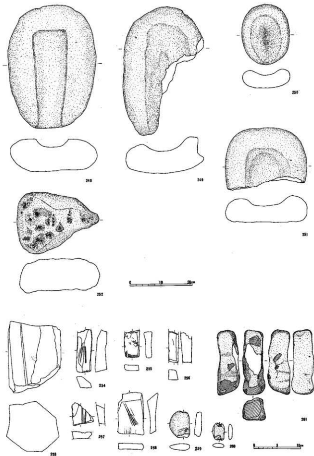
図84 船靈社遺跡縄文・平安時代石器実測図(248~252 1:6、他1:4)
