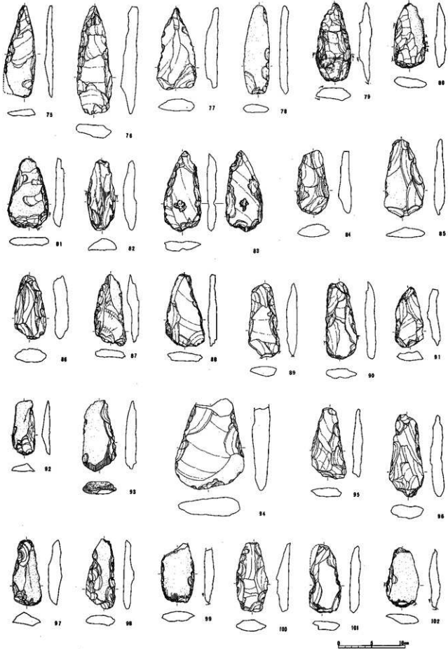
图78 船雲社遺跡縄文時代石器実測図(1:4)
