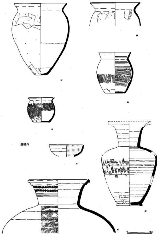
図91 船靈社遺跡平安時代土器実測図(1:4)
