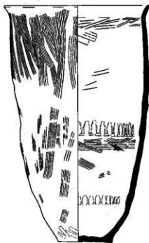
图90 船靈社遺跡平安時代土器実測图 (1:4)
