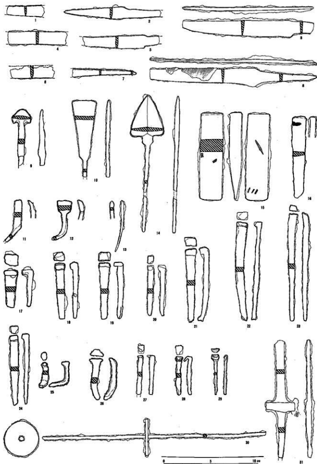
図92 船靈社遺跡平安時代鉄製品実測図(1:2)
