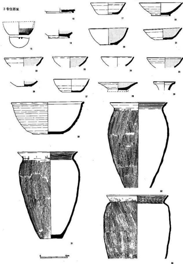
图88 船靈社遺跡平安時代土器実測図(1:4)
