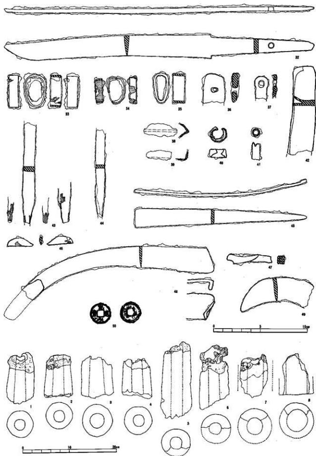
図93 船倉遺跡平安時代鉄製品、土製品実測図 (32-50 1:2、他は1:4)
