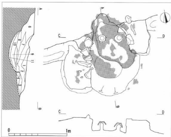
第27図 榎垣外遺跡十王堂地籍1号住居跡カマド平面図(1:20)
