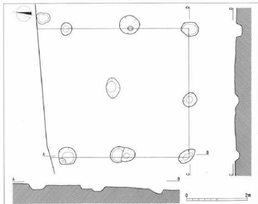
第14図 山道端地籍掘立柱建物跡 (1:60)
