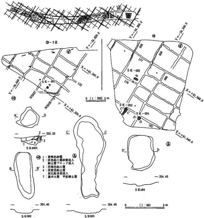
第238図 平安水田土坑 平面・断面 (S K 001-004)
