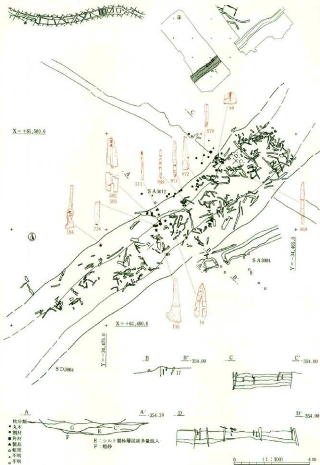
第136図 S D 3004 (①-2区) 平面・断面・立面・出土主要遺物分布図
