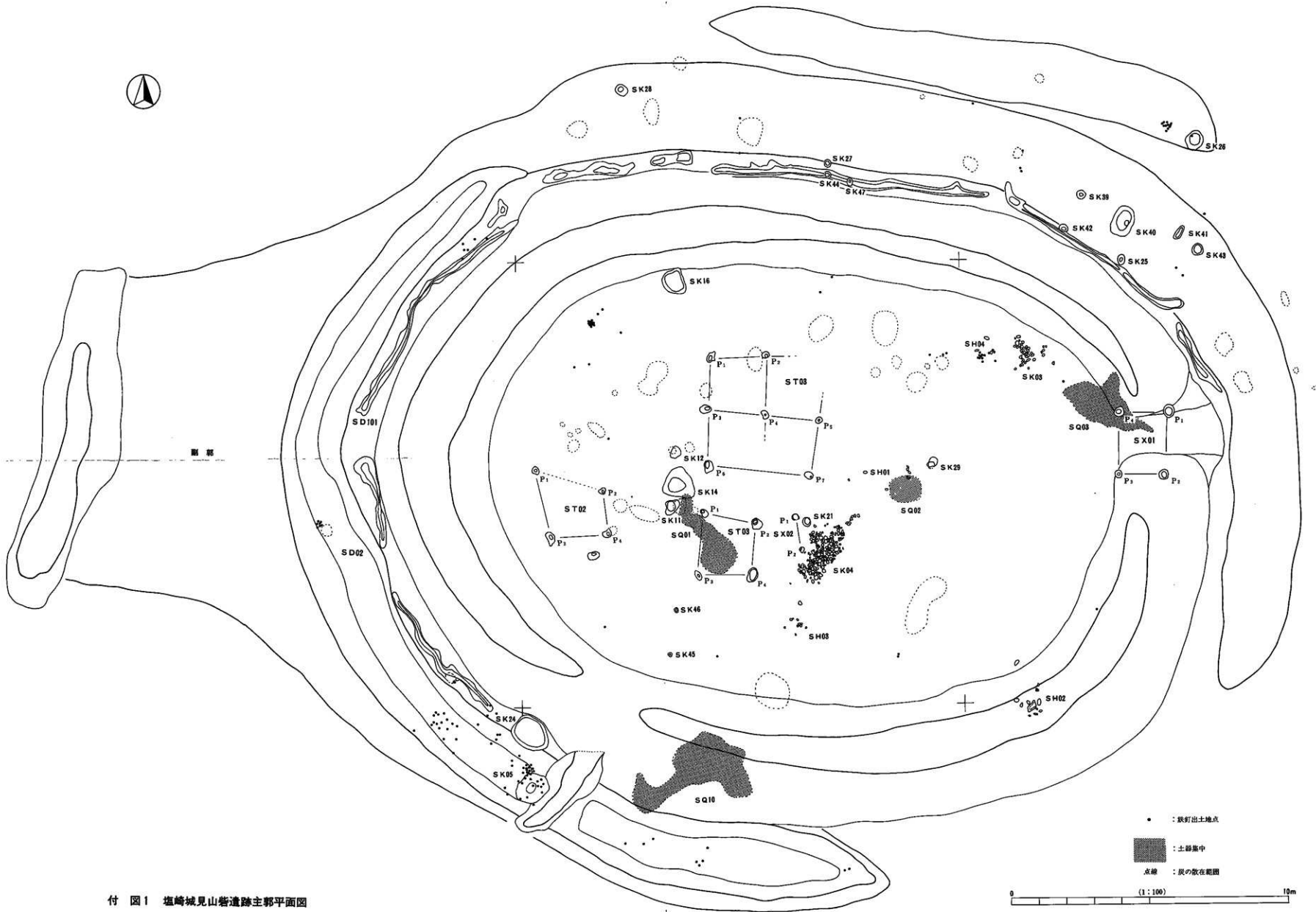
付 図 1 塩崎城見山砦遺跡主郭平面図
