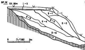
図13 2区〜4区トレンチ断面図および柱状図
