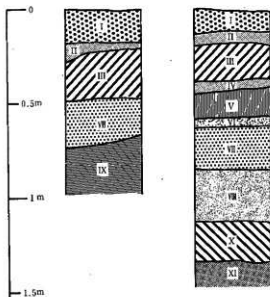
基土層模式図
