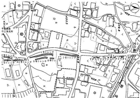
試掘トレンチ設定図 (1:2000)
