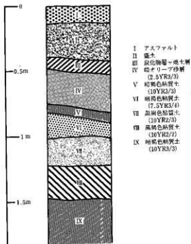
基本土層模式図
