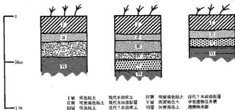
基本土層模式図
