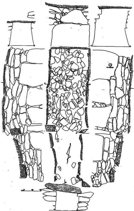
第6圖 神宮寺古墳石室夾測圖1
