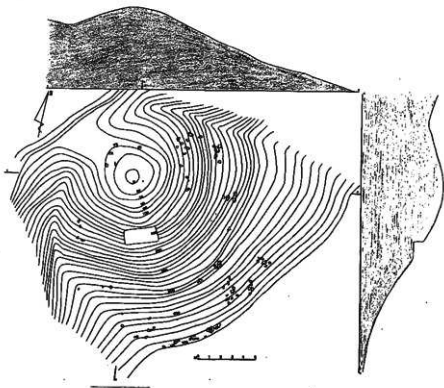
第4図 神宮寺古墳・墳丘実測図
